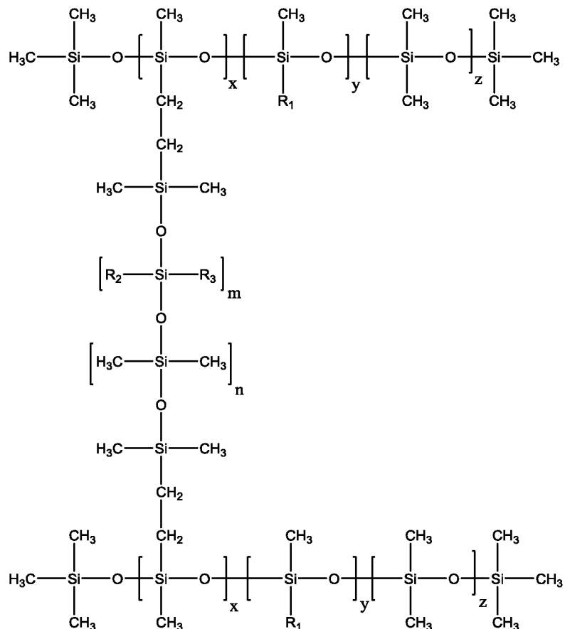
Формула (I)
