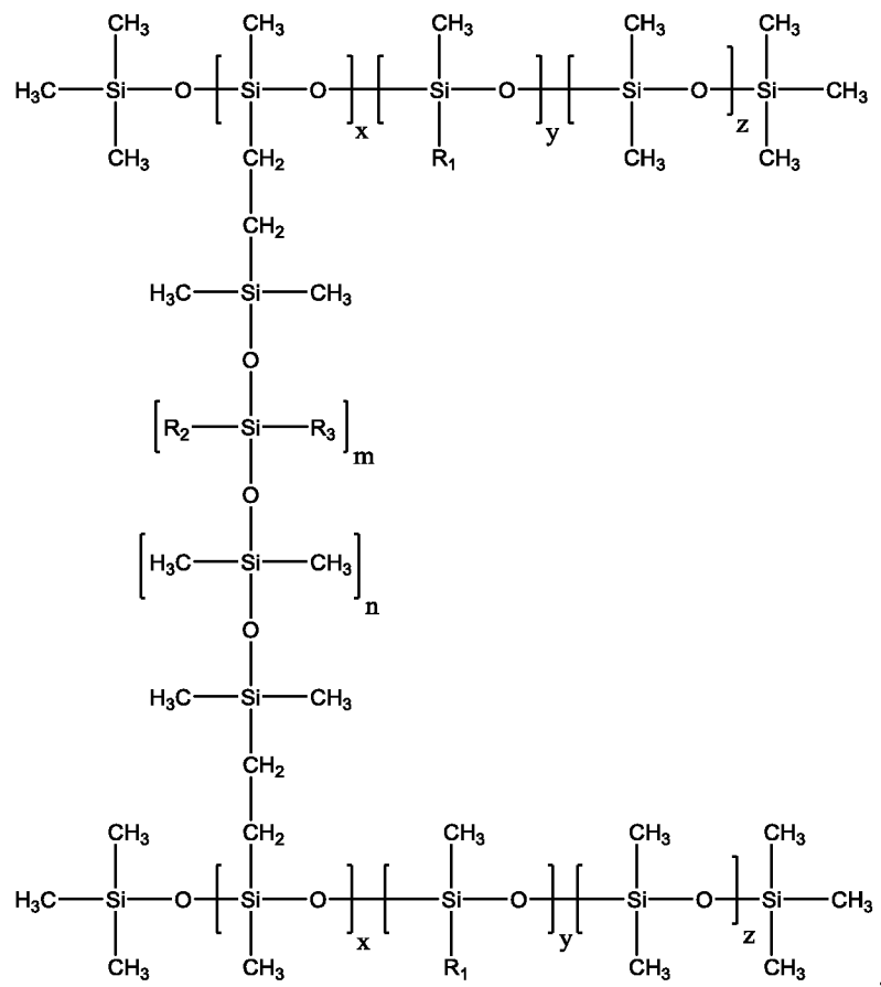
Формула (I)
