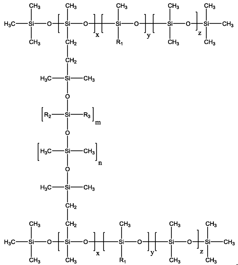
Формула (IV)
