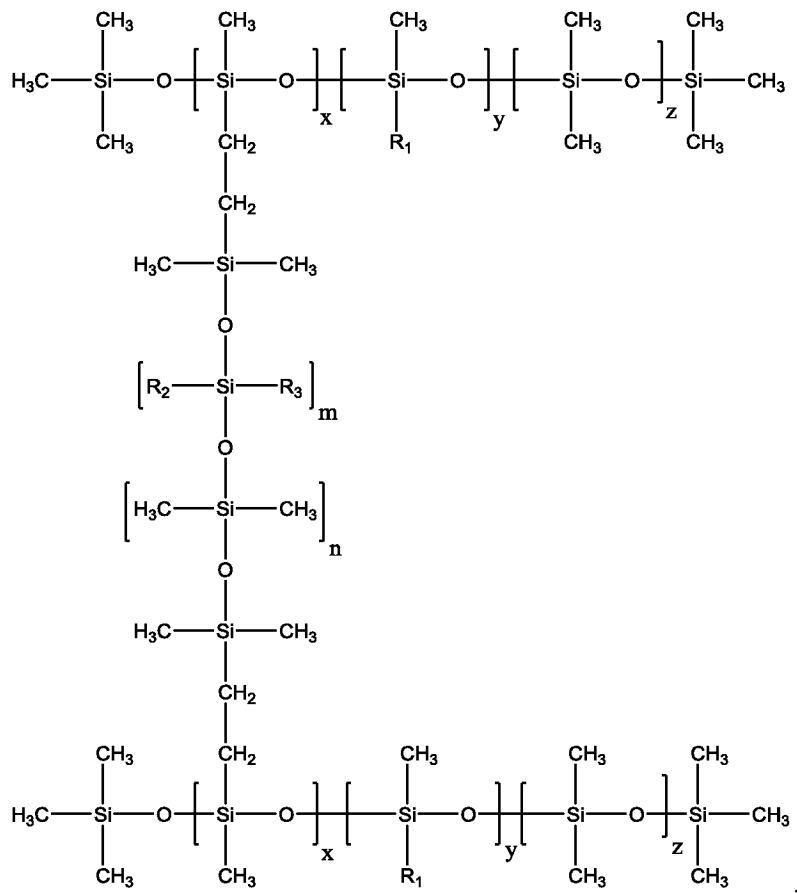
Формула (I)
