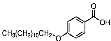
4-(Додэцилокси)бензойная кислота
