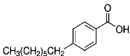
4-Гептилбензойная кислота
