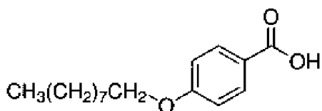
4-(Нонилокси)бензойная кислота
