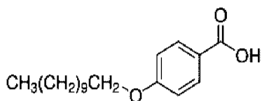
4-(Ундецилокси)бензойная кислота
