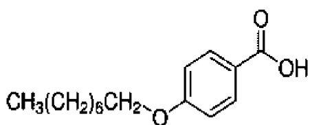
4-(Октилокси)бензойная кислота
