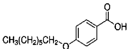
4-(Гептилокси)бензойная кислота
