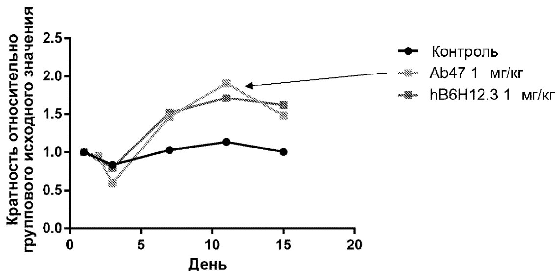
Тромбоциты (Кратность относительно исходного значения) Ab47 в сравнении с hB6H13.3
