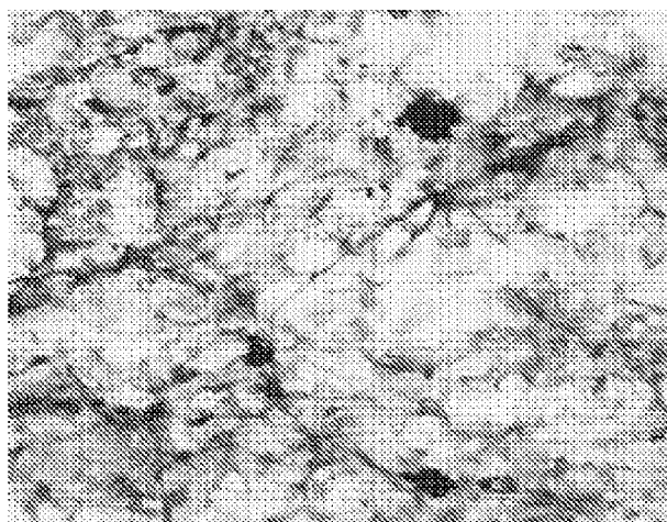
Макрофаг Мыши (детекция с помощью F4/80)
