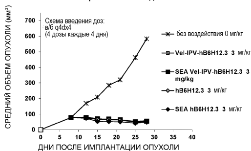
Противоопухолевая активность SEA-направленных антител против CD47 в модели Detroit562
