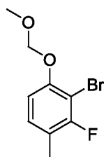
2-бром-3-фтор-1-(метоксиметокси)-4-метилбензол
