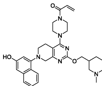
1-(4-(7-(3-гидрокси-1-нафтил)-5,6,7,8-тетрагидропиридо[3,4-d]пиримидин-4-ил)пиперазин-1-ил)проп-2-ен-1-он
