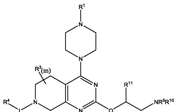
Формула II-A
