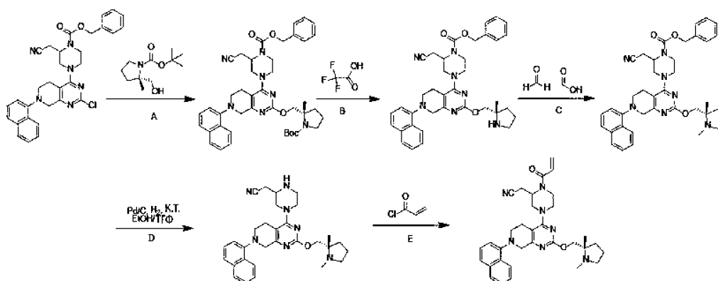
2-(1-акрилоил-4-(2-(((S)-1,2-диметилпирролидин-2-ил)метокси)-7-(нафтален-1-ил)-5,6,7,8-тетрагидропиридо[3,4-d]пиримидин-4-ил)пиперазин-2-ил)ацетонитрил
