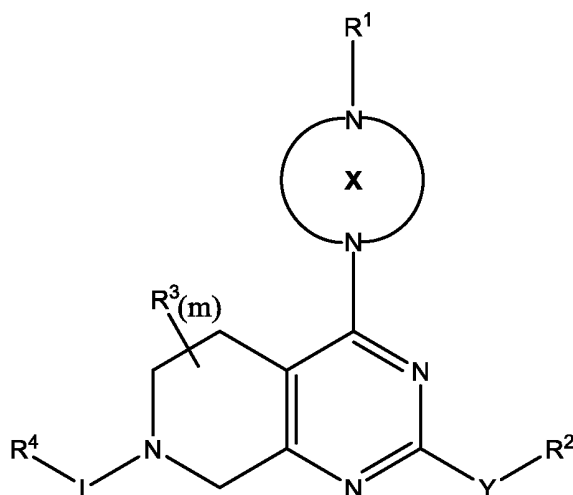
Формула (I)
