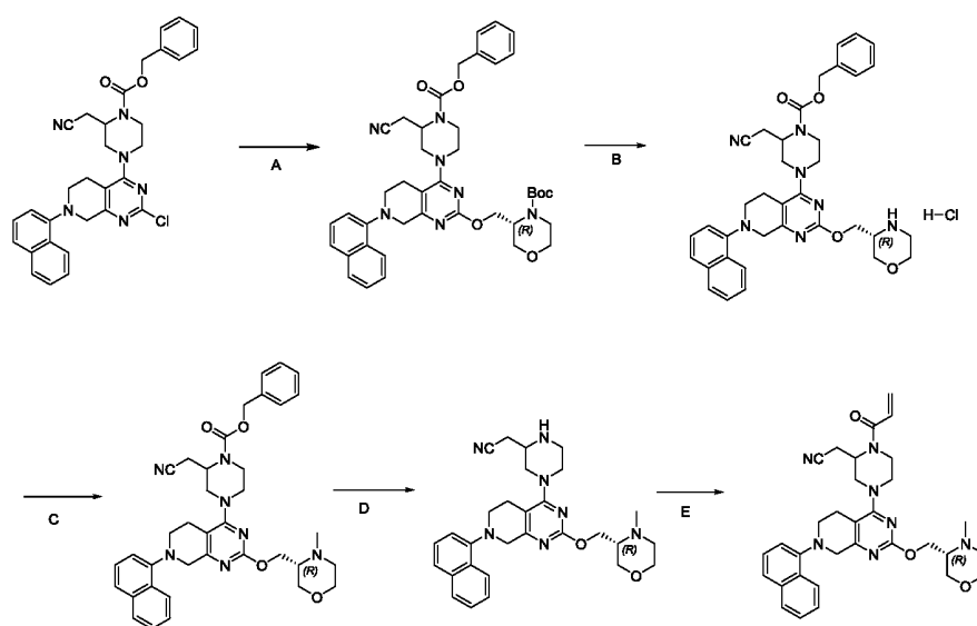
2-(1-Акрилоил-4-(2-(((R)-4-метилморфолин-3-ил)метокси)-7-(нафтален-1-ил)-5,6,7,8-тетрагидропиридо[3,4-d]пиримидин-4-ил)пиперазин-2-ил)ацетонитрил
