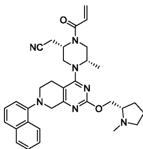
2-((2S,5S)-1-акрилоил-5-метил-4-(2-(((S)-1-метилпирролидин-2-ил)метокси)-7-(нафтален-1-ил)-5,6,7,8-тетрагидропиридо[3,4-d]пиримидин-4-ил)пиперазин-2-ил)ацетонитрил
