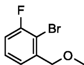
2-бром-1-фтор-3-(метоксиметил)бензол
