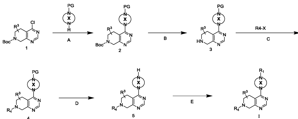
СХЕМА I
