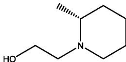
(R)-2-(2-метилпиперидин-1-ил)этан-1-ол
