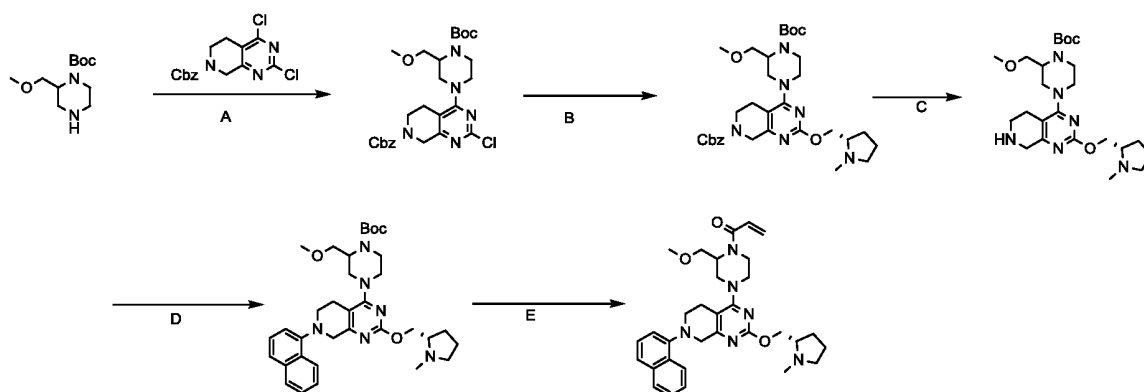
1-(2-(метоксиметил)-4-(2-(((S)-1-метилпирролидин-2-ил)метокси)-7-(нафтален-1-ил)-5,6,7,8-тетрагидропиридо[3,4-d]пиримидин-4-ил)пиперазин-1-ил)проп-2-ен-1-он
