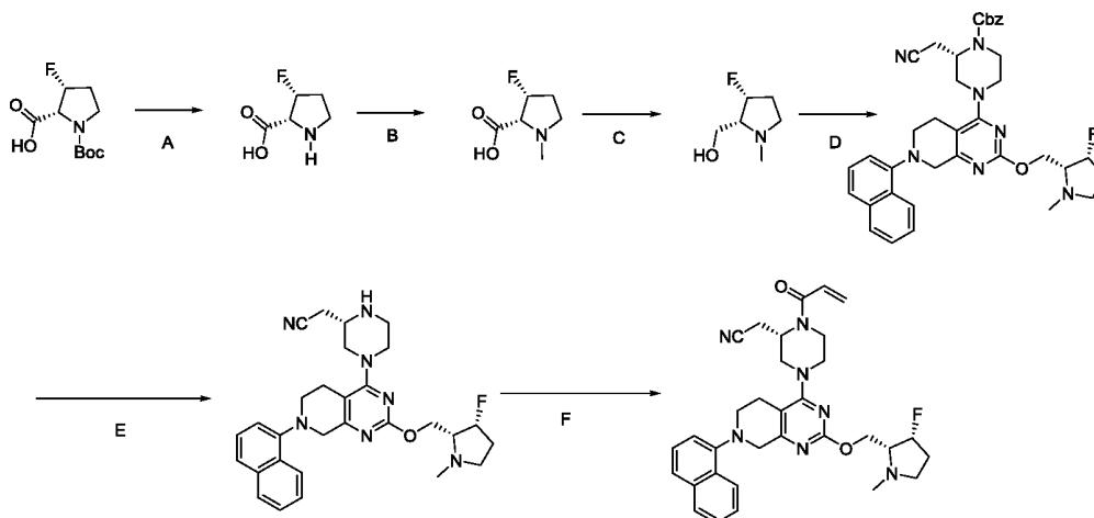
2-((S)-1-акрилоил-4-(2-(((2R,3R)-3-фтор-1-метилпирролидин-2-ил)метокси)-7-(нафтален-1-ил)-5,6,7,8-тетрагидропиrido[3,4-d]пиримидин-4-ил)пиперазин-2-ил)ацетонитрил
