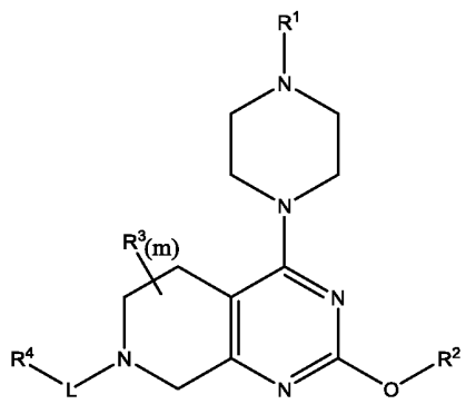
Формула II-B
