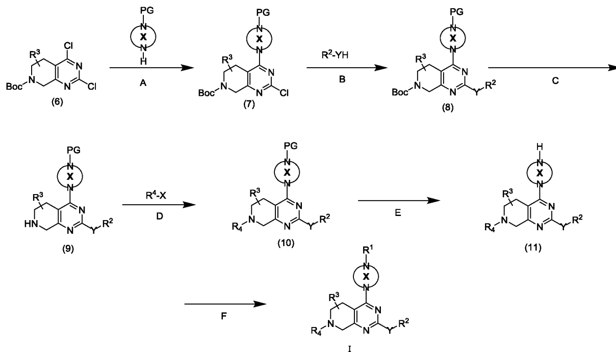
СХЕМА II
