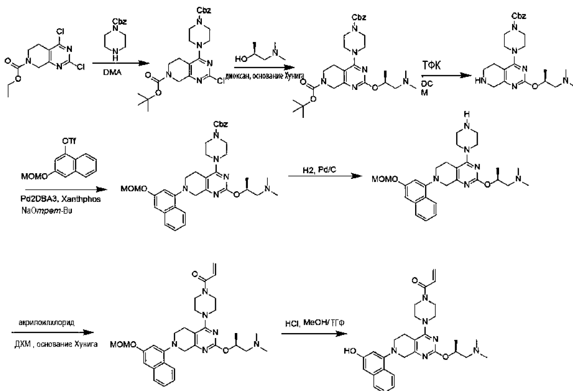
(S)-1-(4-(2-((1-(диметиламино)пропан-2-ил)окси)-7-(3-гидрокси-нафта-1-ил)-5,6,7,8-тетрагидропиридо[3,4-d]пиримидин-4-ил)пиперазин-1-ил)проп-2-ен-1-он
