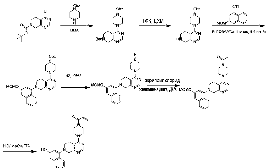
1-(4-(7-(3-гидрокси-1-ил)-5,6,7,8-тетрагидропиридо[3,4-d]пиримидин-4-ил)пиперазин-1-ил)проп-2-ен-1-он
