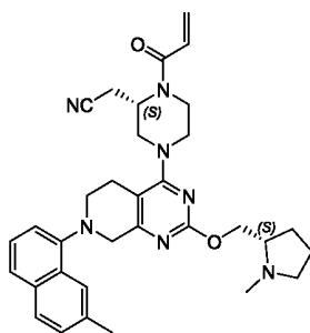
2-((( S )-1-акрилоил-4-(7-(7-метилнафтален-1-ил)-2-((( S )-1-метилпирролидин-2-ил)метокси)-5,6,7,8-тетрагидропиридо[3,4- d ]пиримидин-4-ил)пиперазин-2-ил)ацетонитрил
