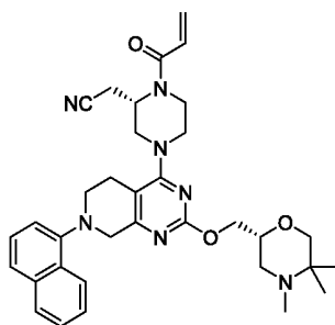
2-((S)-1-Акрилоил-4-(7-(нафтаген-1-ил)-2-(((R)-4,5,5-триметилморфолин-2-ил)метокси)-5,6,7,8-тетрагидропиридо[3,4-d]пиримидин-4-ил)пиперазин-2-ил)ацетонитрил
