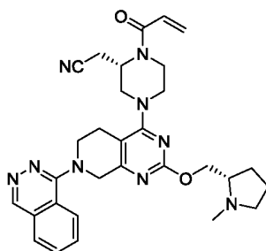
2-((S)-1-акрилоил-4-(2-(((S)-1-метилпирролидин-2-ил)метокси)-7-(фталазин-1-ил)-5,6,7,8-тетрагидропиридо[3,4-d]пиримидин-4-ил)пиперазин-2-ил)ацетонитрил
