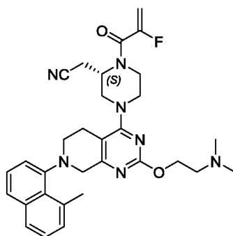
2-[(2S)-4-[2-[2-(Диметиламино)этокси]-7-(8-метил-1-нафтил)-6,8-дигидро-5H-пиридо[3,4-d]пиримидин-4-ил]-1-(2-фторпроп-2-еноил)пиперазин-2-ил]ацетонитрил
