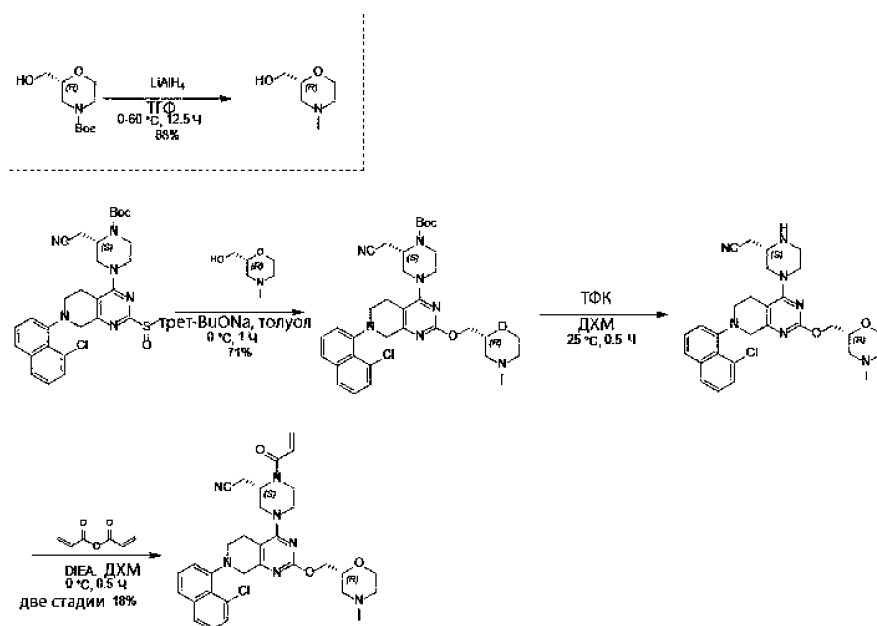
2-[(2S)-4-[7-(8-хлор-1-нафтил)-2-[[[(2R)-4-метилморфолин-2-ил]метокси]-6,8-дигидро-5H-пиридо[3,4-d]пиримидин-4-ил]-1-проп-2-еноил-пиперазин-2-ил]ацетонитрил
