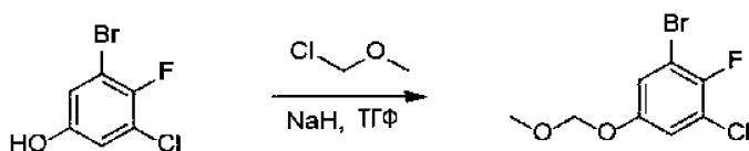
1-бром-3-хлор-2-фтор-5-(метоксиметокси)бензол
