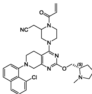
2-(1-акрилоил-4-(7-(8-хлорнафтален-1-ил)-2-((( S )-1-метилпирролидин-2-ил)метокси)-5,6,7,8-тетрагидропиридо[3,4- d ]пиримидин-4-ил)пиперазин-2-ил)ацетонитрил
