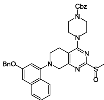
бензил 4-(7-(3-(бензилокси)нафтаден-1-ил)-2-(метилсульфинил)-5,6,7,8-тетрагидропиридо[3,4-d]пиримидин-4-ил)пиперазин-1-карбоксилат
