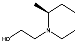
(S)-2-(2-метилпиперидин-1-ил)этан-1-ол
