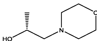
(R)-1-морфолинпропан-2-ол
