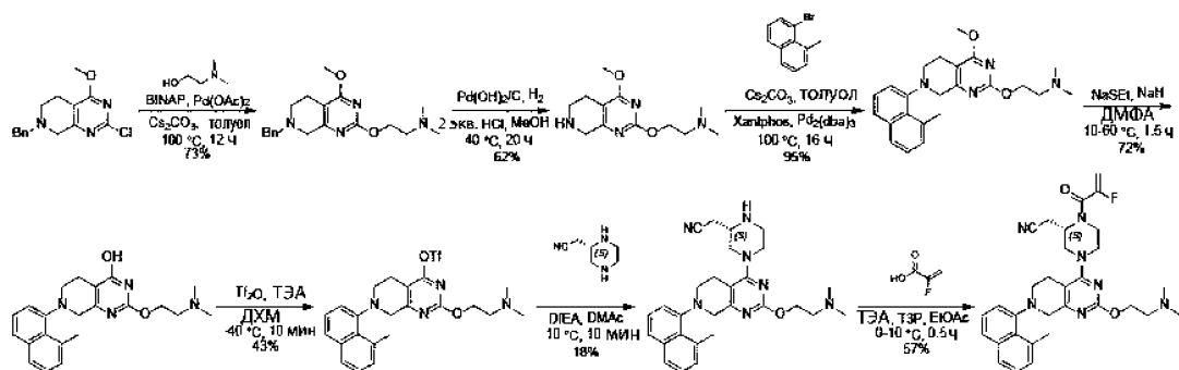
2-[(2S)-4-[2-[2-(Диметиламино)этокси]-7-(8-метил-1-нафтил)-6,8-дигидро-5H-пиридо[3,4-d]пиримидин-4-ил]-1-(2-фторпроп-2-еноил)пиперазин-2-ил]ацетонитрил
