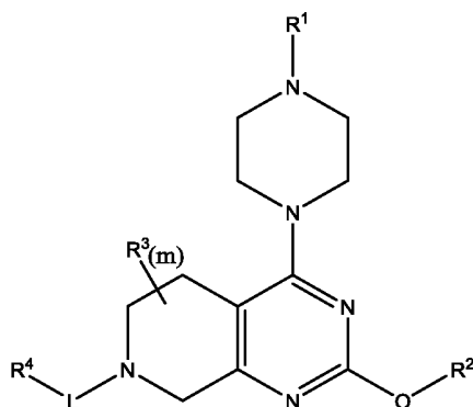
Формула I-B
