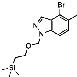
4-бром-5-метил-1-((2-(триметилсилил)этокс)метил)-1H-индазол
