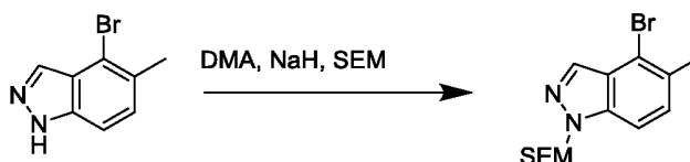
4-бром-5-метил-1-((2-(триметилсилил)этокс)метил)-1H-индазол
