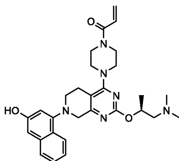
(S)-1-(4-(2-((1-(диметиламино)пропан-2-ил)окси)-7-(3-гидрокси-нафта-1-ил)-5,6,7,8-тетрагидропиридо[3,4-d]пиримидин-4-ил)пиперазин-1-ил)проп-2-ен-1-он
