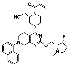
2-((S)-1-акрилоил-4-(2-(((2R,3R)-3-фтор-1-метилпирролидин-2-ил)метокси)-7-(нафтален-1-ил)-5,6,7,8-тетрагидропиrido[3,4-d]пиримидин-4-ил)пиперазин-2-ил)ацетонитрил
