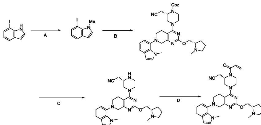
2-((S)-1-акрилоил-4-(7-(1-метил-1H-индол-7-ил)-2-(((S)-1-метилпирролидин-2-ил)метокси)-5,6,7,8-тетрагидропиридо[3,4-d]пиримидин-4-ил)пиперазин-2-ил)ацетонитрил
