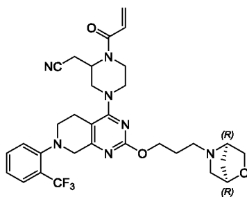
2-(1-акрилоил-4-(2-((( R )-1-метилпирролидин-3-ил)метокси)-7-(2-(трифторметил)фенил)-5,6,7,8-тетрагидропиридо[3,4- d ]пиримидин-4-ил)пиперазин-2-ил)ацетонитрил
