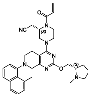
2-((( S )-1-акрилоил-4-(7-(8-метилнафтаген-1-ил)-2-((( S )-1-метилпирролидин-2-ил)метокси)-5,6,7,8-тетрагидропиридо[3,4- d ]пиримидин-4-ил)пиперазин-2-ил)ацетонитрил
