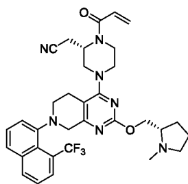
2-(((S)-1-акрилоил-4-(2-(((S)-1-метилпирролидин-2-ил)метокси)-7-(8-(трифторметил)нафтален-1-ил)-5,6,7,8-тетрагидропиридо[3,4-d]пиримидин-4-ил)пиперазин-2-ил)ацетонитрил
