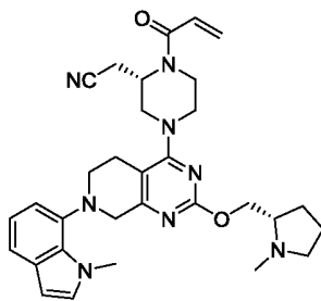
2-((S)-1-акрилоил-4-(7-(1-метил-1H-индол-7-ил)-2-(((S)-1-метилпирролидин-2-ил)метокси)-5,6,7,8-тетрагидропиридо[3,4-d]пиримидин-4-ил)пиперазин-2-ил)ацетонитрил
