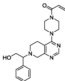
1-(4-(7-(2-гидрокси-1-фенилэтил)-5,6,7,8-тетрагидропиридо[3,4-d]пиримидин-4-ил)пиперазин-1-ил)проп-2-ен-1-он
