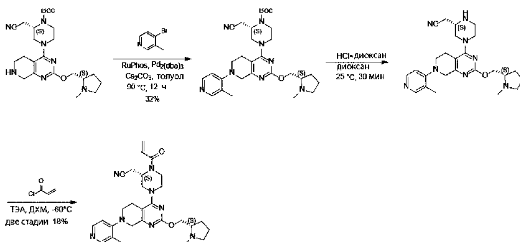
2-[(2 S )-4-[7-(3-метил-4-пиридил)-2-[[[(2 S )-1-метилпирролидин-2-ил]метокси]-6,8-дигидро-5 H -пиридо[3,4- d ]пиримидин-4-ил]-1-проп-2-еноил-пиперазин-2-ил]ацетонитрил
