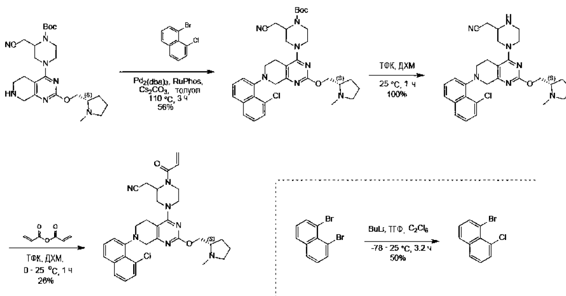
2-(1-акрилоил-4-(7-(8-хлорнафтален-1-ил)-2-((( S )-1-метилпирролидин-2-ил)метокси)-5,6,7,8-тетрагидропиридо[3,4- d ]пиримидин-4-ил)пиперазин-2-ил)ацетонитрил
