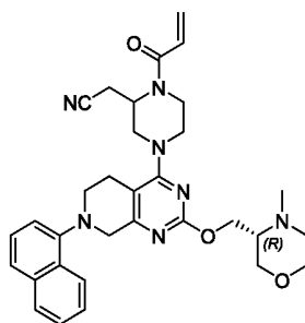
2-(1-Акрилоил-4-(2-(((R)-4-метилморфолин-3-ил)метокси)-7-(нафтален-1-ил)-5,6,7,8-тетрагидропиридо[3,4-d]пиримидин-4-ил)пиперазин-2-ил)ацетонитрил
