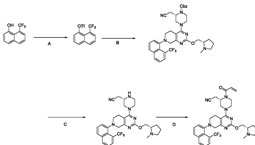
2-(((S)-1-акрилоил-4-(2-(((S)-1-метилпирролидин-2-ил)метокси)-7-(8-(трифторметил)нафтален-1-ил)-5,6,7,8-тетрагидропиридо[3,4-d]пиримидин-4-ил)пиперазин-2-ил)ацетонитрил
