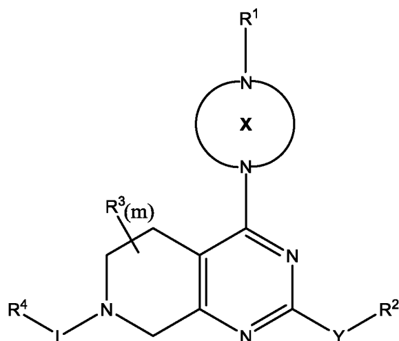
Формула (I)
