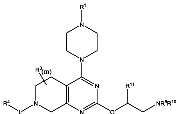
Формула I-A
