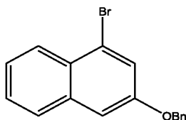
4-бромнафтален-2-ол
