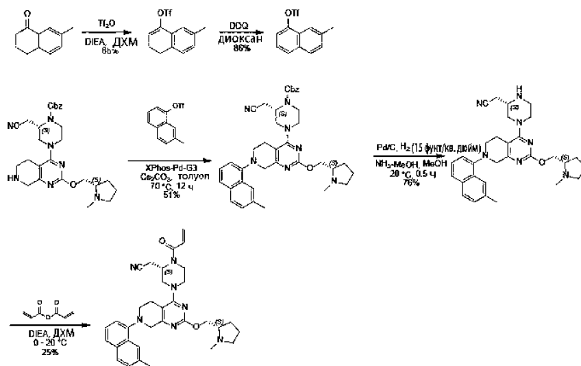
2-((( S )-1-акрилоил-4-(7-(7-метилнафтален-1-ил)-2-((( S )-1-метилпирролидин-2-ил)метокси)-5,6,7,8-тетрагидропиридо[3,4- d ]пиримидин-4-ил)пиперазин-2-ил)ацетонитрил
