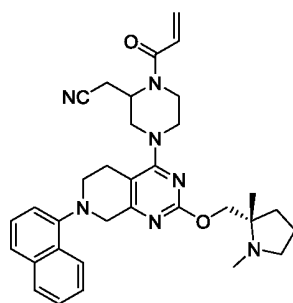
2-(1-акрилоил-4-(2-(((S)-1,2-диметилпирролидин-2-ил)метокси)-7-(нафтален-1-ил)-5,6,7,8-тетрагидропиридо[3,4-d]пиримидин-4-ил)пиперазин-2-ил)ацетонитрил
