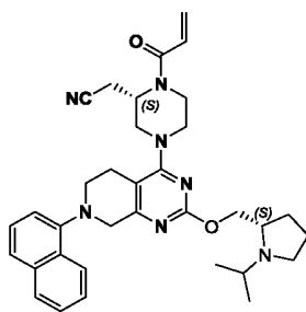
2-[(2 S )-4-[2-[[[(2 S )-1-изопропилпирролидин-2-ил]метокси]-7-(1-нафтил)-6,8-дигидро-5 H -пиридо[3,4- d ]пиримидин-4-ил]пиперазин-2-ил]ацетонитрил
