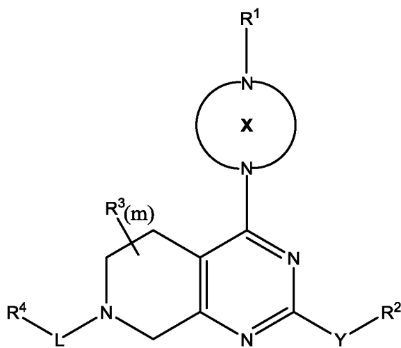
Формула (II)
