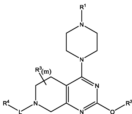
Формула II-B
