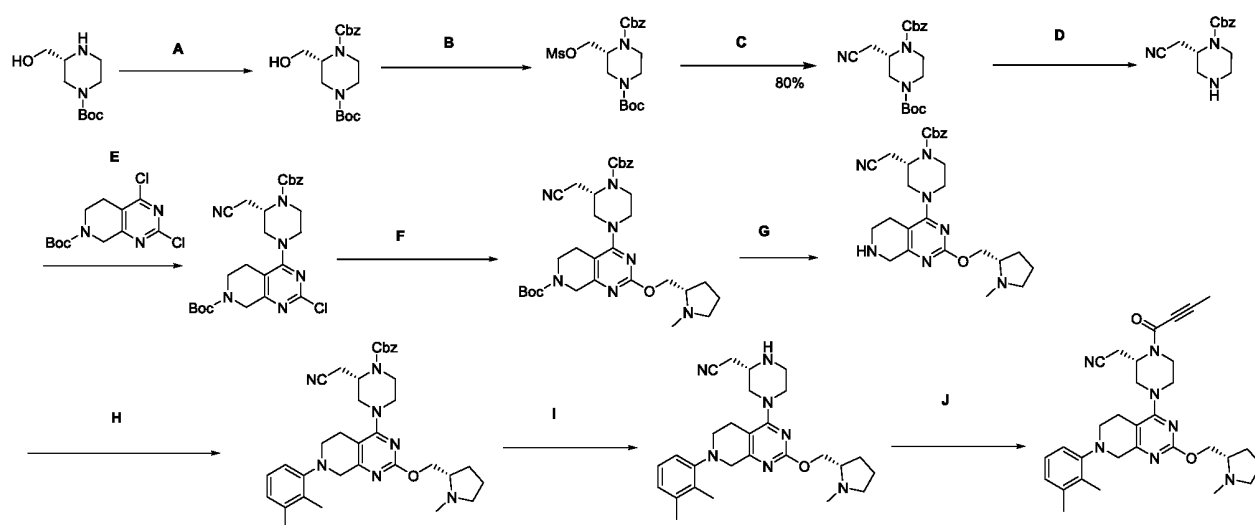
2-(((S)-1-(бют-2-иноил)-4-(7-(2,3-диметилфенил)-2-(((S)-1-метилпирролидин-2-ил)метокси)-5,6,7,8-тетрагидропиридо[3,4-d]пиримидин-4-ил)пиперазин-2-ил)ацетонитрил
