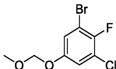
1-бром-3-хлор-2-фтор-5-(метоксиметокси)бензол
