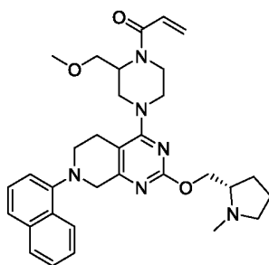
1-(2-(метоксиметил)-4-(2-(((S)-1-метилпирролидин-2-ил)метокси)-7-(нафтален-1-ил)-5,6,7,8-тетрагидропиридо[3,4-d]пиримидин-4-ил)пиперазин-1-ил)проп-2-ен-1-он
