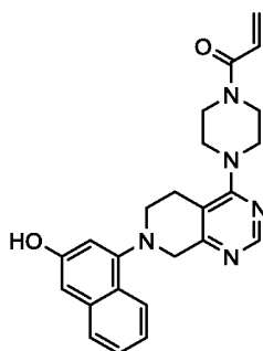
1-(4-(7-(3-гидрокси-1-ил)-5,6,7,8-тетрагидропиридо[3,4-d]пиримидин-4-ил)пиперазин-1-ил)проп-2-ен-1-он
