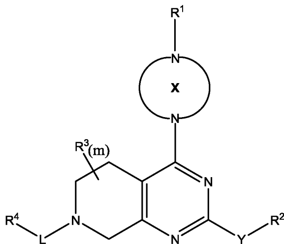
Формула (II)
