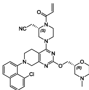
2-[(2S)-4-[7-(8-хлор-1-нафтил)-2-[[[(2R)-4-метилморфолин-2-ил]метокси]-6,8-дигидро-5H-пиридо[3,4-d]пиримидин-4-ил]-1-проп-2-еноил-пиперазин-2-ил]ацетонитрил
