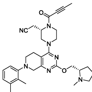
2-(((S)-1-(бют-2-иноил)-4-(7-(2,3-диметилфенил)-2-(((S)-1-метилпирролидин-2-ил)метокси)-5,6,7,8-тетрагидропиридо[3,4-d]пиримидин-4-ил)пиперазин-2-ил)ацетонитрил
