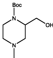
трет-бутил 2-(гидроксиметил)-4-метилпиперазин-1-карбоксилат
