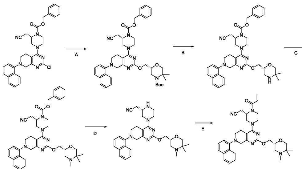
2-((S)-1-Акрилоил-4-(7-(нафтаген-1-ил)-2-(((R)-4,5,5-триметилморфолин-2-ил)метокси)-5,6,7,8-тетрагидропиридо[3,4-d]пиримидин-4-ил)пиперазин-2-ил)ацетонитрил
