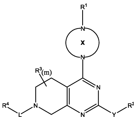
Формула (II)
