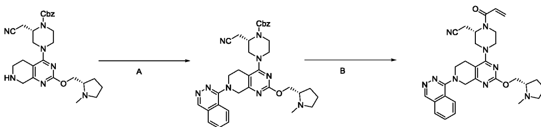
2-((S)-1-акрилоил-4-(2-(((S)-1-метилпирролидин-2-ил)метокси)-7-(фталазин-1-ил)-5,6,7,8-тетрагидропиридо[3,4-d]пиримидин-4-ил)пиперазин-2-ил)ацетонитрил
