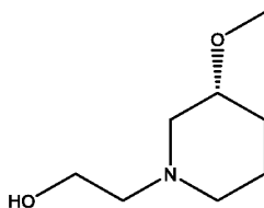
(R)-2-(3-метоксипиперидин-1-ил)этан-1-ол
