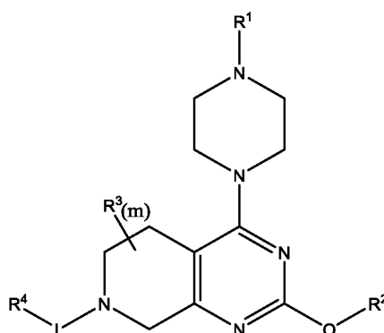
Формула II-B
