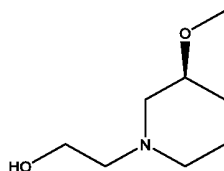
(S)-2-(3-метоксипиперидин-1-ил)этан-1-ол
