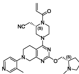
2-[(2 S )-4-[7-(3-метил-4-пиридил)-2-[[[(2 S )-1-метилпирролидин-2-ил]метокси]-6,8-дигидро-5 H -пиридо[3,4- d ]пиримидин-4-ил]-1-проп-2-еноил-пиперазин-2-ил]ацетонитрил
