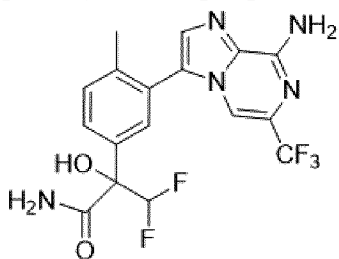
Стадия 1. 1-(3-бром-4-метилфенил)-2,2-дифторэтан-1-ол
