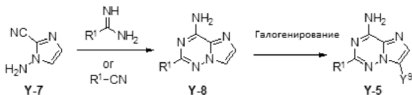
Схема Y-B.
