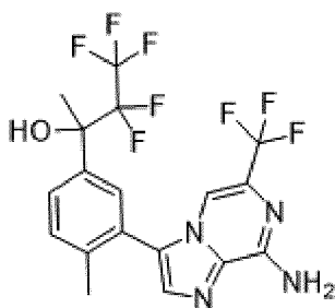
Стадия 1. 2-(3-бром-4-метилфенил)-3,3,4,4,4-пентафторбутан-2-ол
