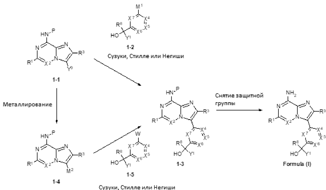
Схема I.
