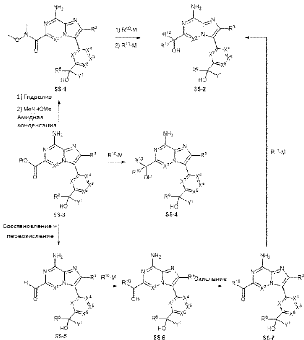
Схема XXIX.
