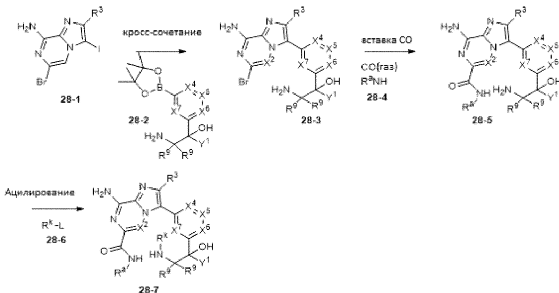
Схема XXVIII.
