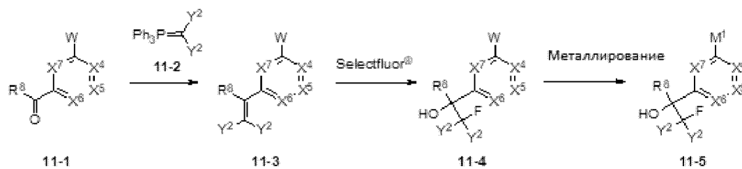
Схема XI.
