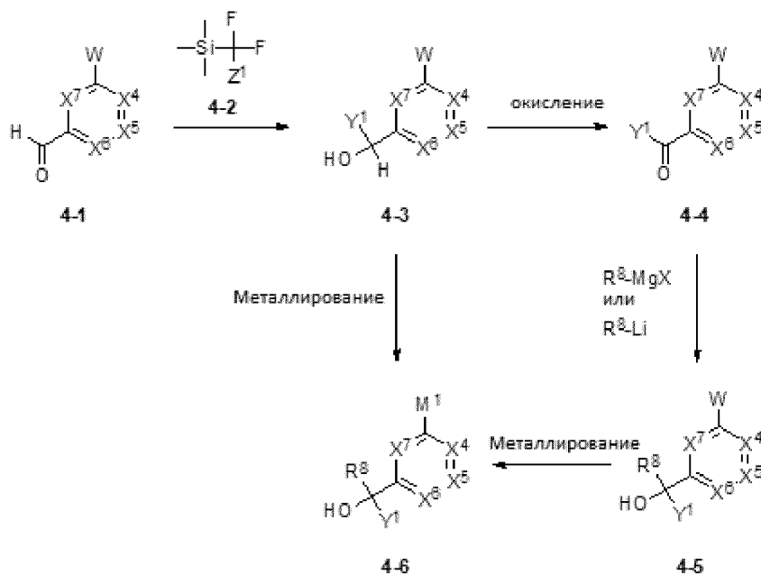
Схема IV.
