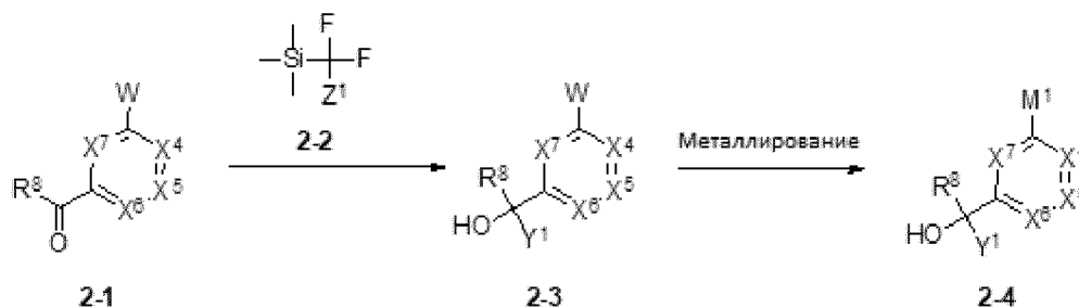
Схема II.
