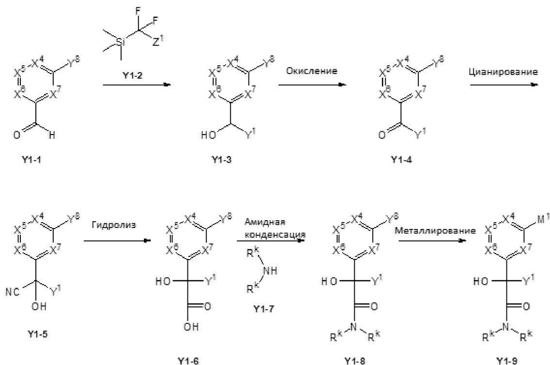
Схема Y1.
