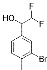
Стадия 1. 1-(3-бром-4-метилфенил)-2,2-дифторэтан-1-ол
