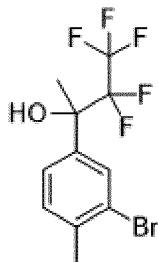
Стадия 1. 2-(3-бром-4-метилфенил)-3,3,4,4,4-пентафторбутан-2-ол
