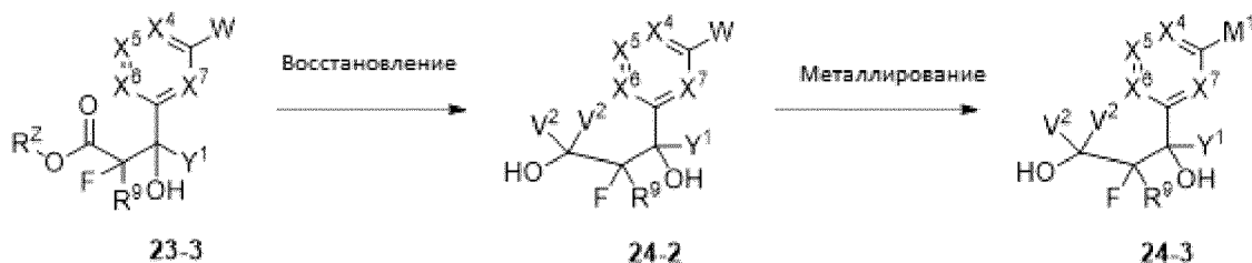
Схема XXIV.
