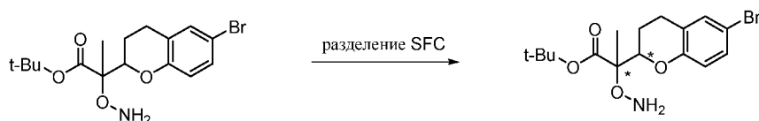
4 стереоизомера: I-1a, I-1b, I-1c, I-1d
