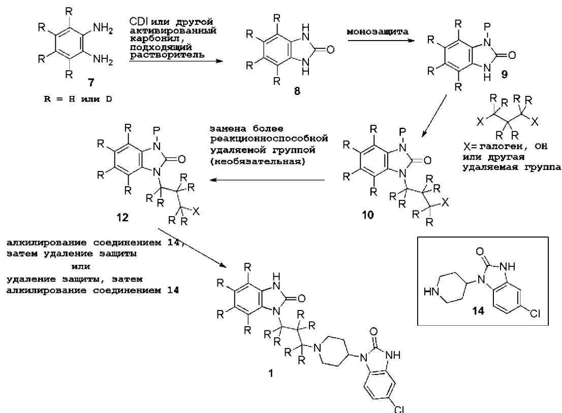
Схема 1: Общий синтез дейтерированного домперидона
