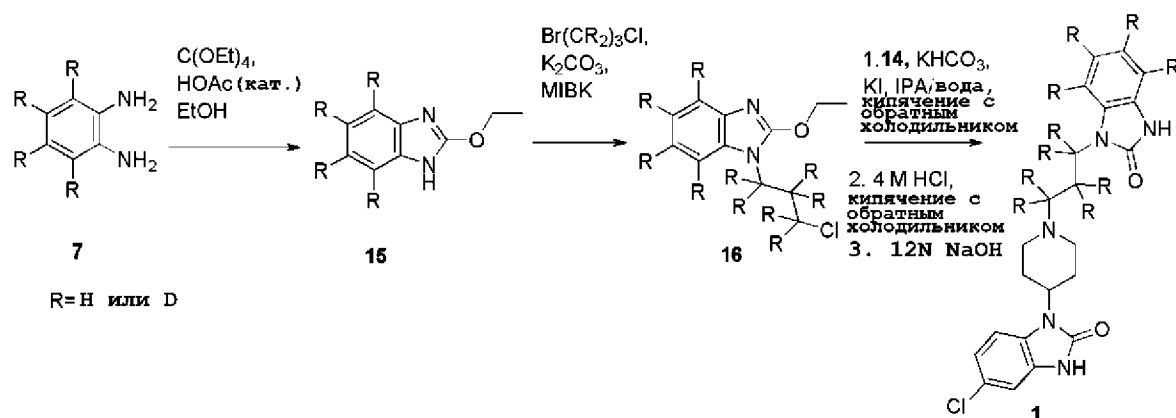
Схема 2 Синтез дейтерированного домперидона
