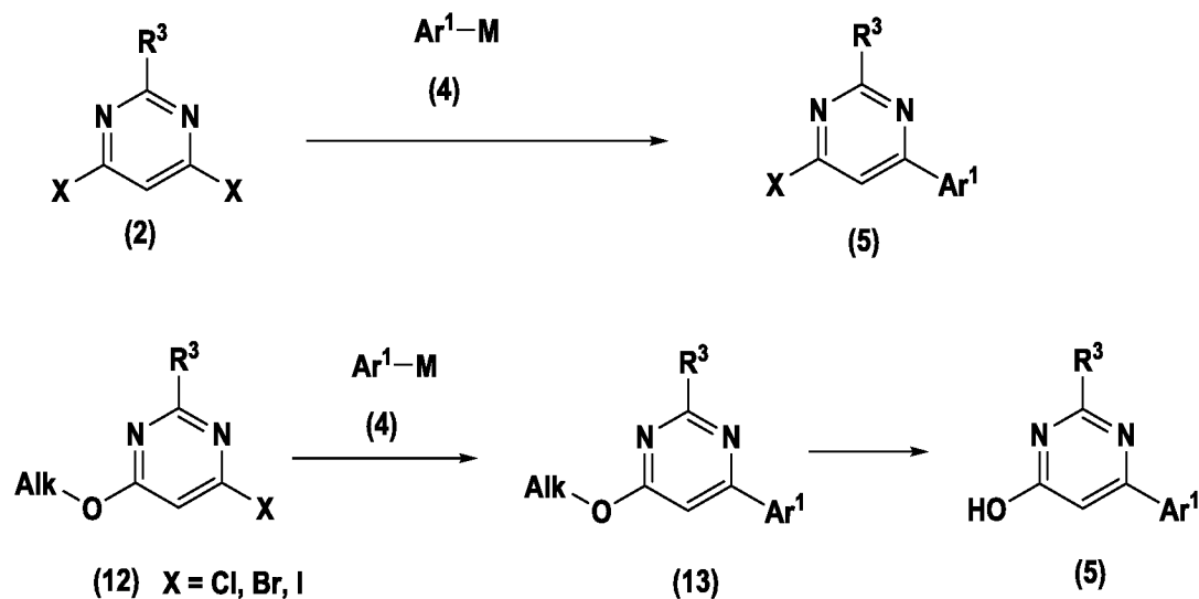
Схема 3. Получение пиримидинов (5)
