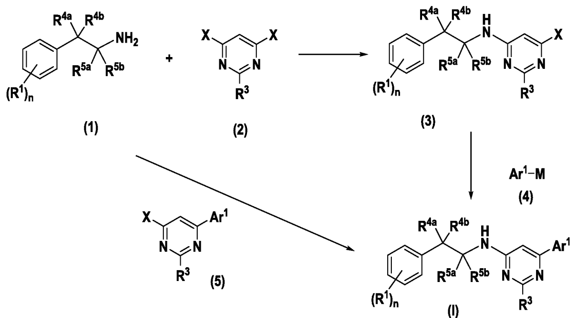
Схема 1: Общие пути получения соединений формулы (I)
