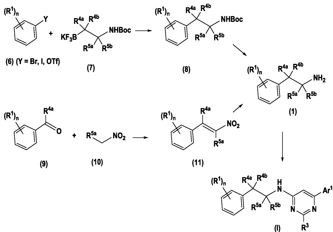
Схема 2. Получение замещенных β-аминоэтил-ароматических соединений (1)
