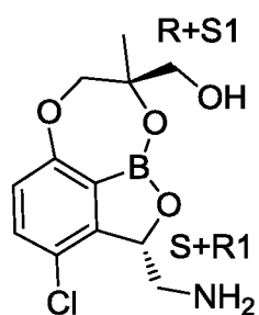
Пример 14
