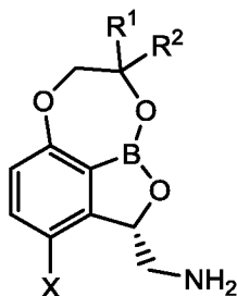
Формула IIa,
