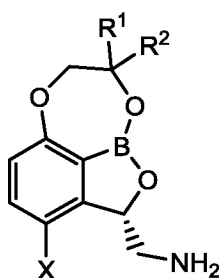
Формула IIa,
