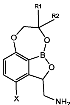
Формула II,
