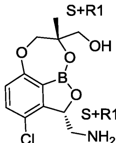
Пример 15
