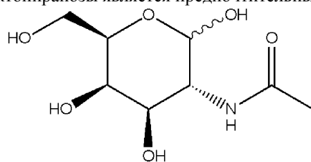
2-(Ацетиламино)-2-дезоксид-D-галактопираноза
