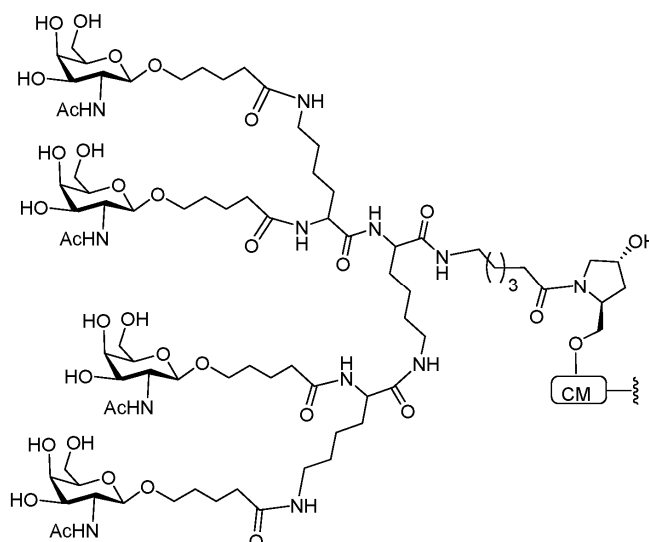
Пример 51. Получение олигонуклеотида 155, содержащего GalNAc 3 -6
