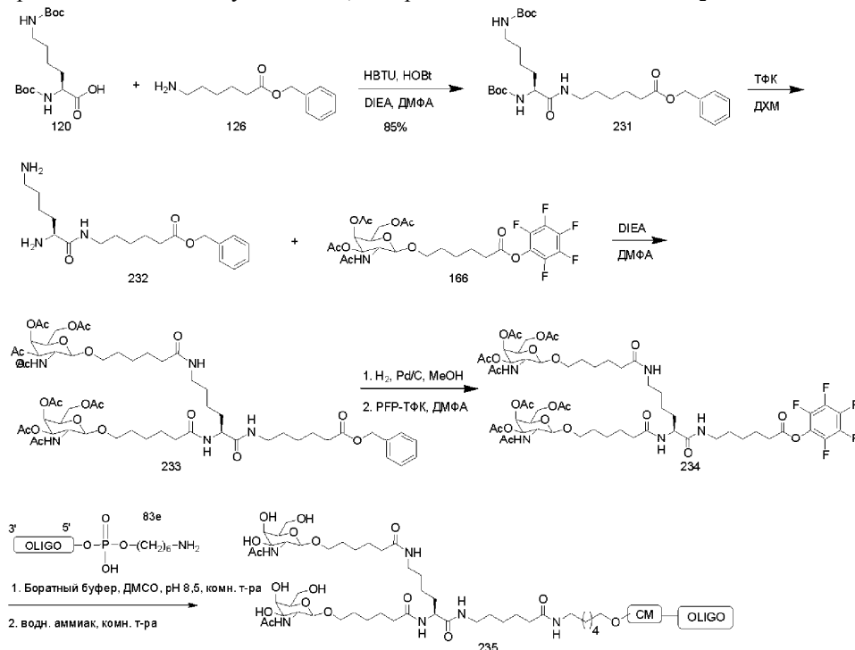
Пример 104. Синтез олигонуклеотидов, содержащих конъюгат 5'-GalNAc 2 .
