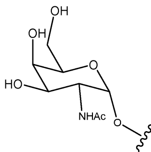
2-(Ацетиламино)-2-дезоксид- \alpha -D-галактопираноза
