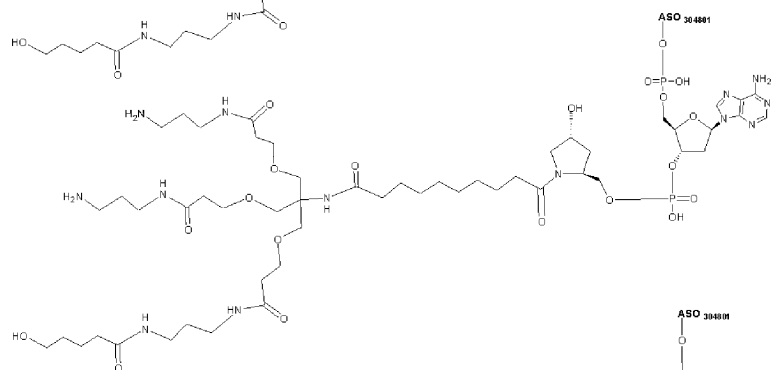
Метаболит 5
