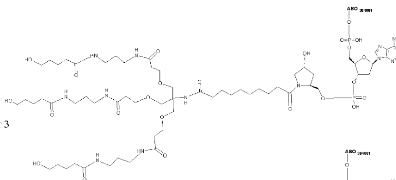
Метаболит 2
