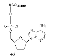
Метаболит 2
