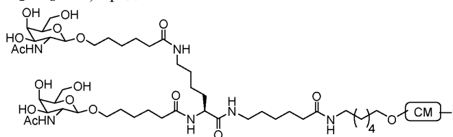
Пример 105. Синтез олигонуклеотидов, содержащих конъюгат GalNAc 1 -25
