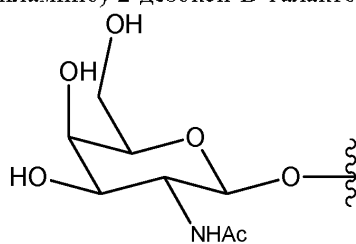
2-(Ацетиламино)-2-дезоксид-D-галактопираноза
