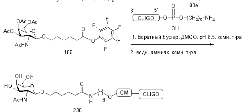
Пример 105. Синтез олигонуклеотидов, содержащих конъюгат GalNAc 1 -25
