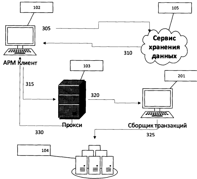
Распределенная база данных с неизменяемыми параметрами Фиг. 3
