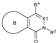
Формула (XV)
