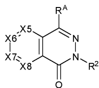
Формула (V)
