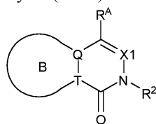
Формула (XXII)
