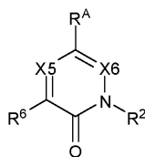
Формула (VIIa)
