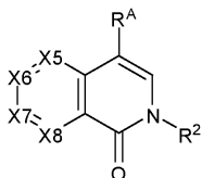
Формула (XII)
