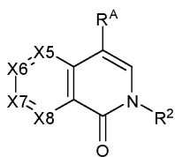
Формула (Ib)
