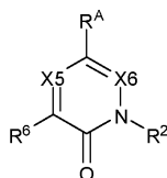
Формула (VII)
