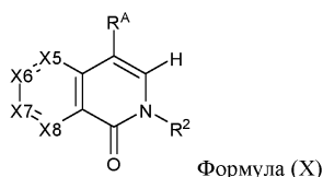
Формула (X)
