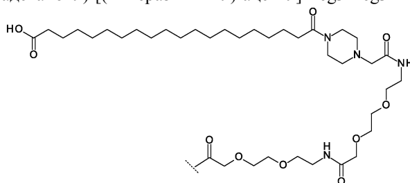
(xiii) (19-карбоксононадеканоил)-[(пиперазин-1-ил)-ацетил]-Peg6
