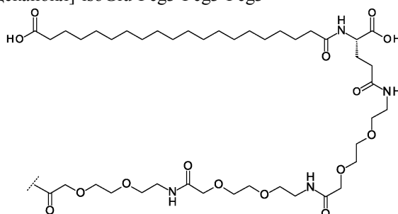
(xi) [19-карбоксононадеканоил]-isoGlu-Peg3-Peg3
