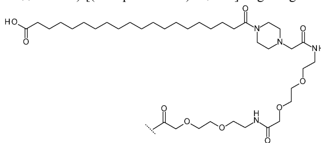
(xii) (19-Карбокси-нонадеcanoил)-[(пиперазин-1-ил)-ацетил]-Peg3-Peg3
