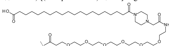
(xiii) (19-карбоксихептадеcanoил)-[(пиперазин-1-ил)ацетил]-Peg6
