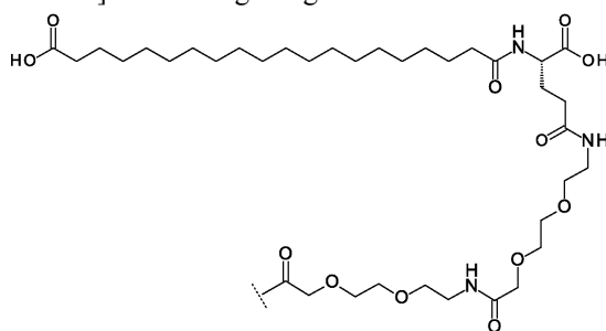
(xii) (19-карбоксононадеканоил)-[(пиперазин-1-ил)-ацетил]-Peg3-Peg3
