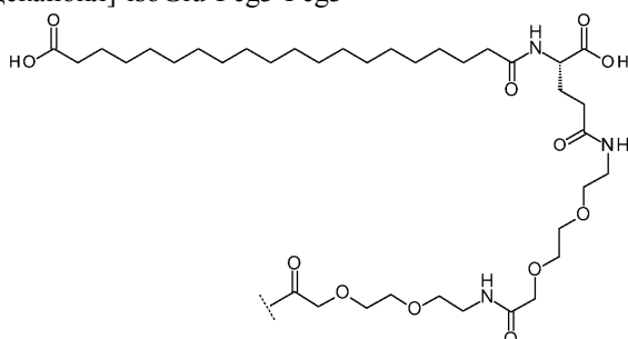
(xii) (19-Карбокси-нонадеcanoил)-[(пиперазин-1-ил)-ацетил]-Peg3-Peg3
