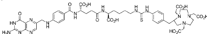
EC1778 C 45 H 57 N 13 O 13 S Точная масса: 1019,39 Мол. вес: 1020,08
