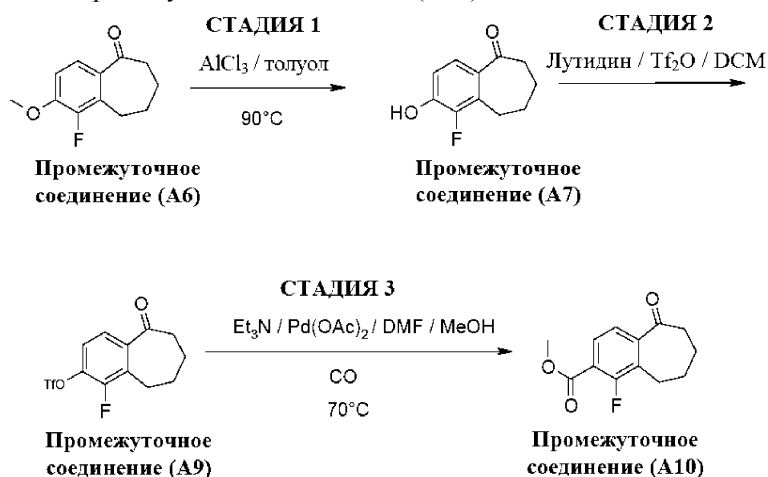
Схема 3. Получение промежуточного соединения (A10)
