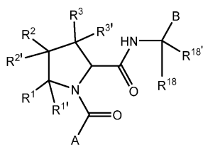
Формула III
