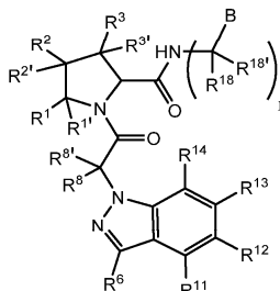
Формула XVIII
