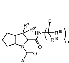
Формула XV
