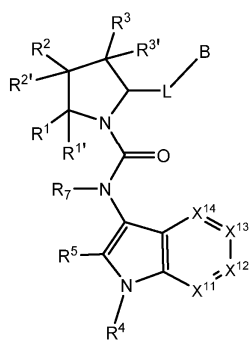
Формула VIII
