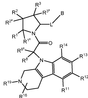
Формула XIII
