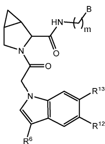
Формула XXVII
