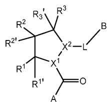
Формула II
