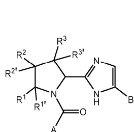
Формула V
