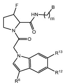
Формула XXVI
