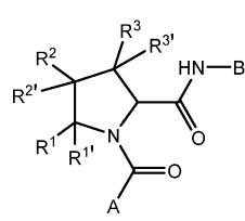
Формула IV
