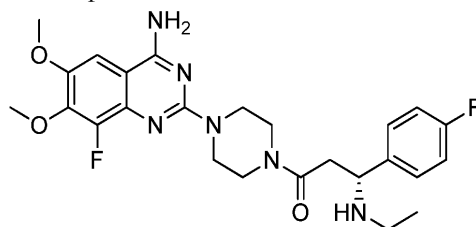
Структура ингибитора фактора В комплемента
