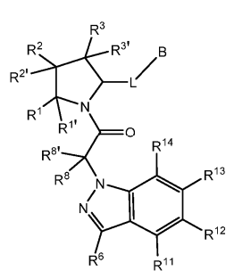
Формула XI
