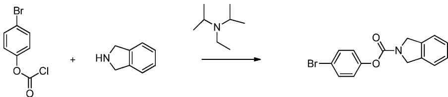
Пример 68А. 4-Бромфенил изоиндолин-2-карбоксилат
