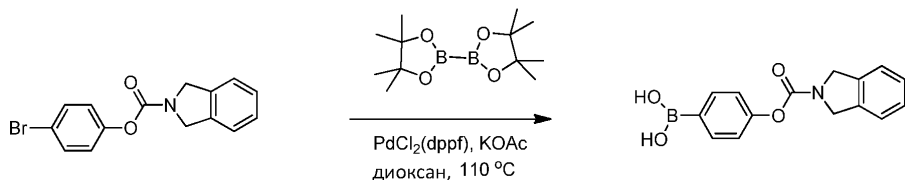
Пример 68В. 4-((Изоиндолин-2-карбонил)окси)фенил)бороновая кислота
