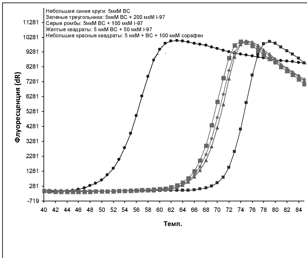
Фигура 2. Результаты исследования теплового сдвига соединения I-97 в отношении домена биотинкарбоксилазы ACC2.
