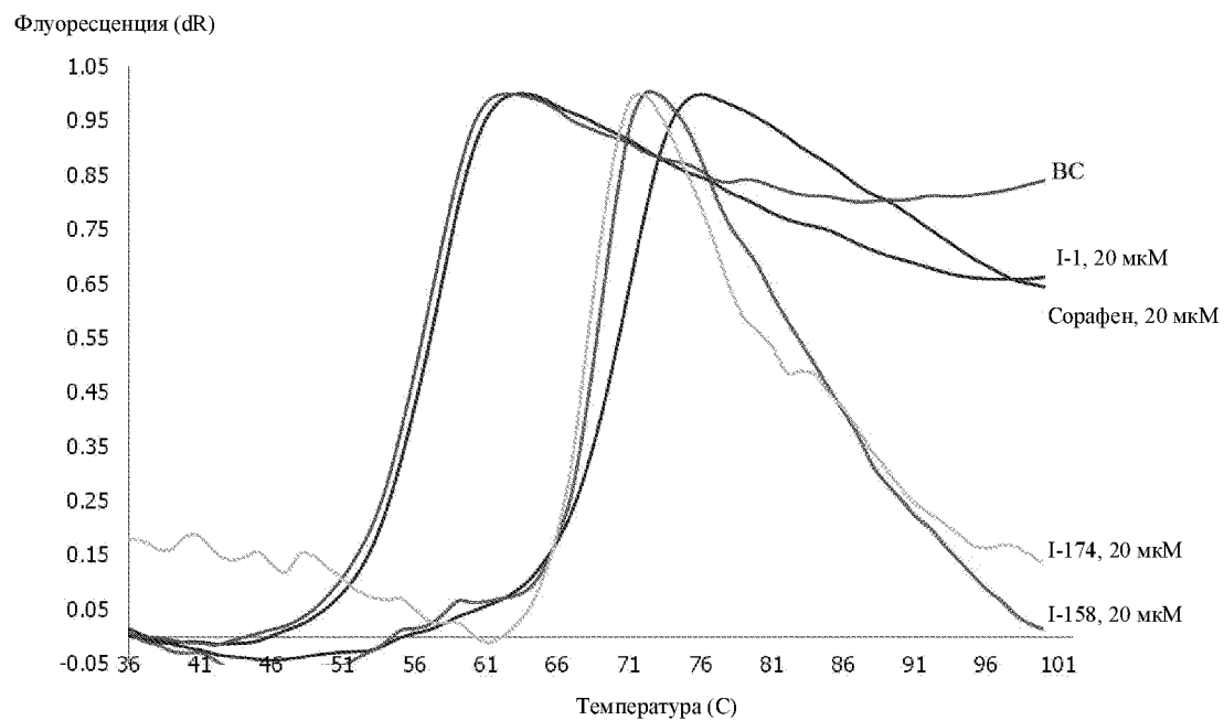
Фигура 3. Результаты исследования теплового сдвига соединений I-1, I-158, I-174 и сорафена А в отношении домена биотинкарбоксилазы ACC2.
