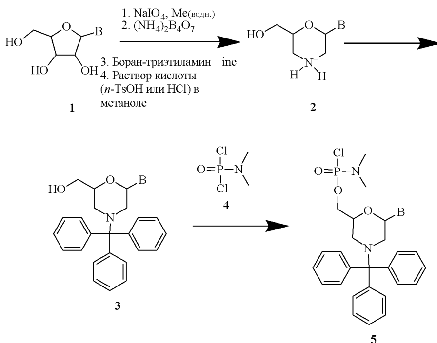
Схема 1: Общий путь синтеза субъединиц РМО
