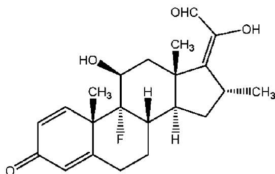
E-изомер енольного альдегида дексаметазона
