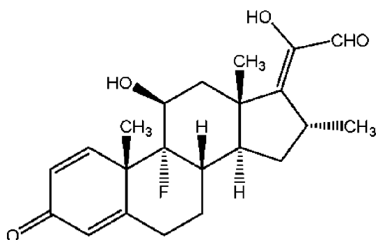
Z-изомер енольного альдегида дексаметазона
