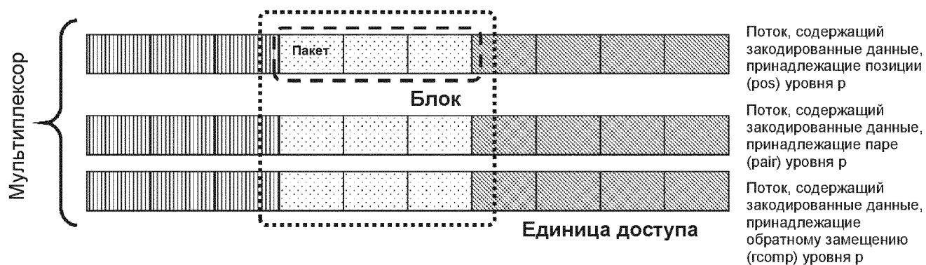
Фигура 26 – Единицы доступа образуются блоками данных, принадлежащими нескольким уровням и индексированным с использованием механизмов MIT и LIT.
