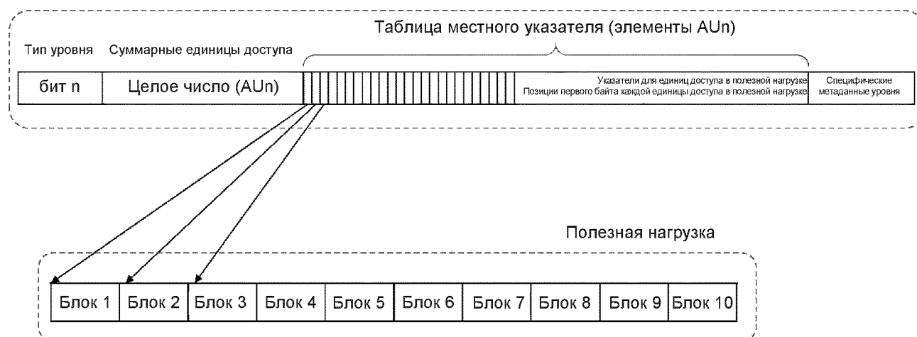
Фигура 23 – Таблица местного указателя в заголовке уровня представляет собой вектор указателей к единицам доступа в полезной нагрузке.
