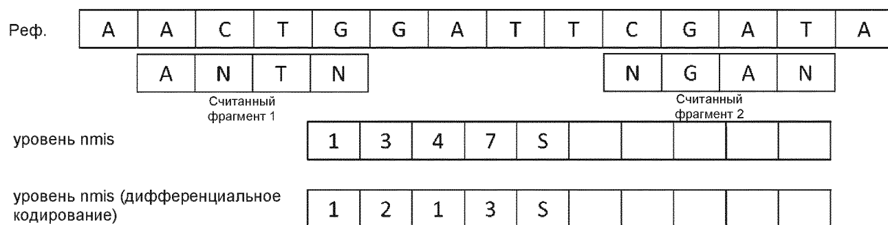
Фигура 11 - Вычисление N рассогласований в уровне nmis.
