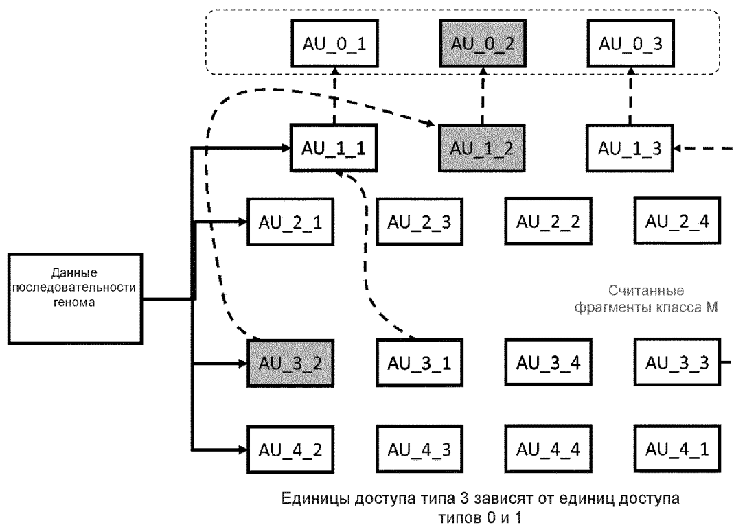
Фигура 39 – Единицы доступа, требуемые для декодирования считанных выборок последовательности с рассогласованиями, подставленными во второй сегмент референсной последовательности (AU 0-2).
