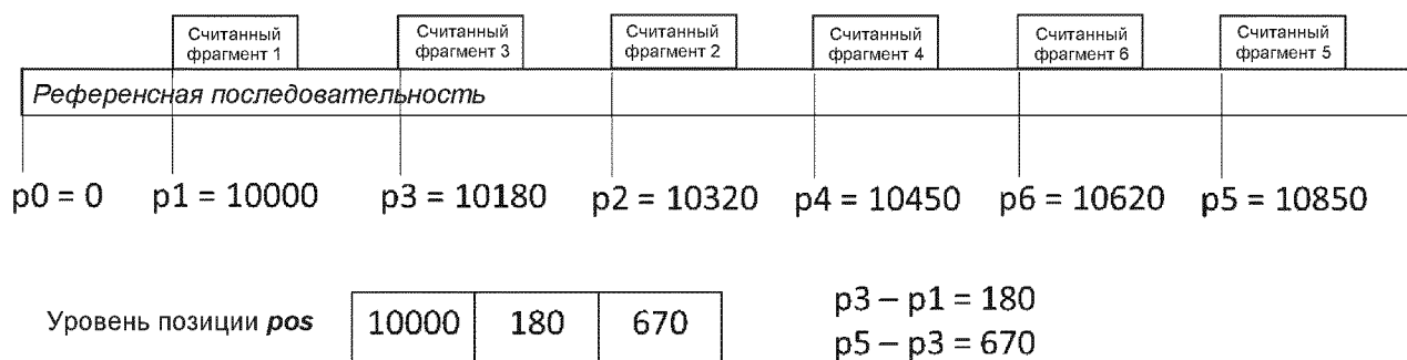
Фигура 4 - Способ отображения и кодирования позиции первого считанного фрагмента из трех пар считанных фрагментов, подставленных и закодированных на уровне позиции ( pos ).
