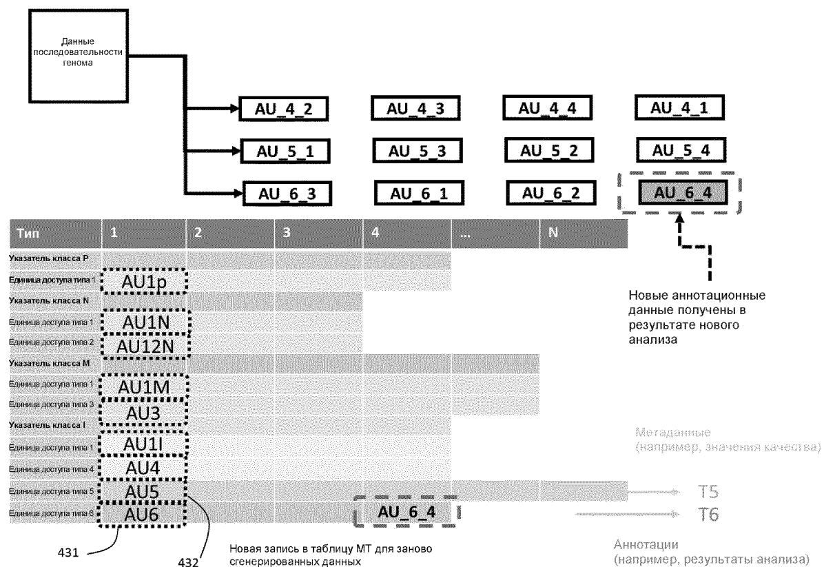
Фигура 43 - Заново полученные результаты анализа инкапсулируются в новую единицу доступа типа 6 и соответствующий индекс создается в таблице Главного указателя.
