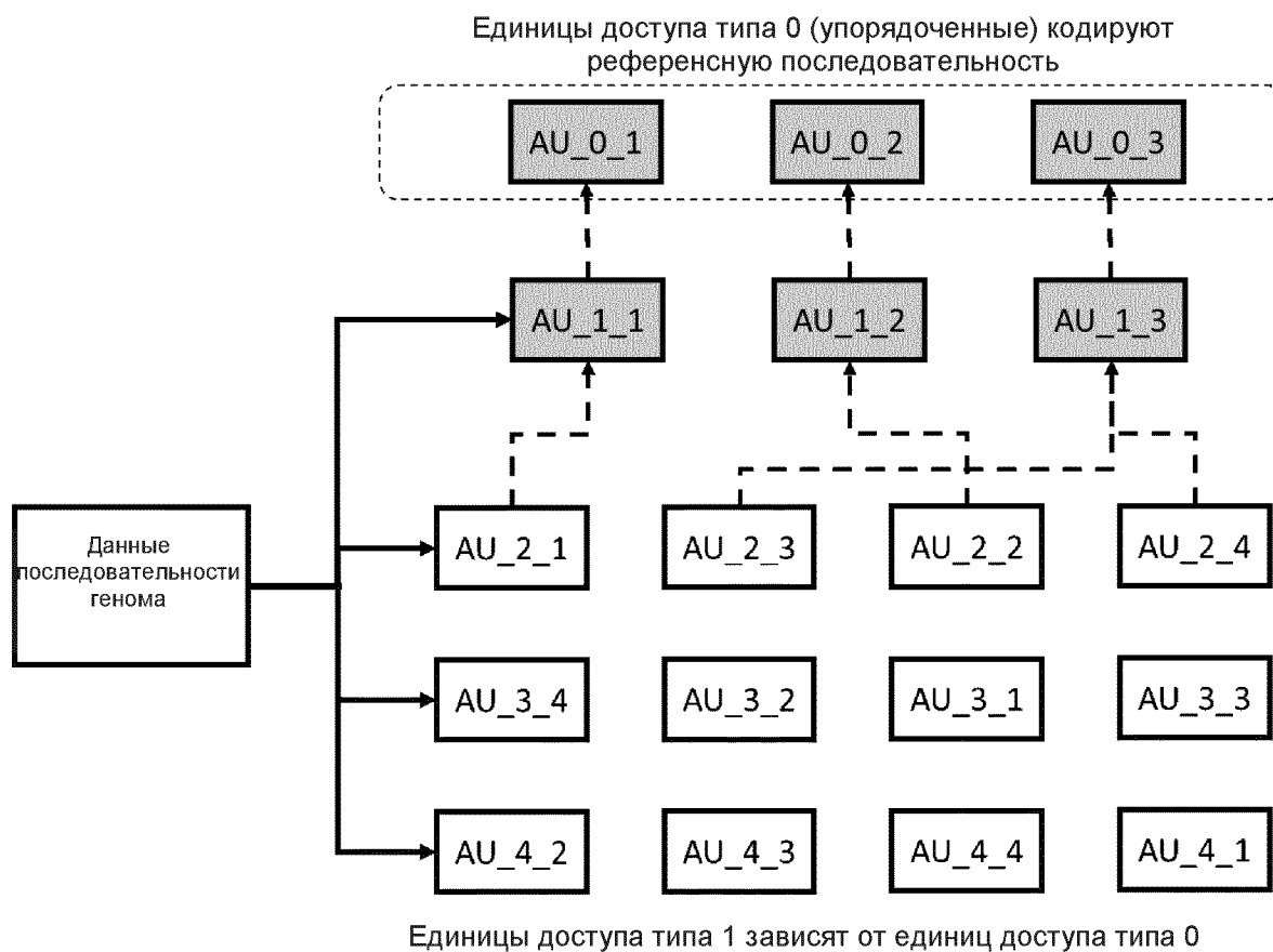
Фигура 35 - Единицы доступа типа 1 соотносятся с требующими декодирования единицами доступа типа 0.
