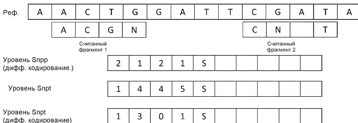
Фигура 15 - Кодирование замен внутри уровня snpt.
