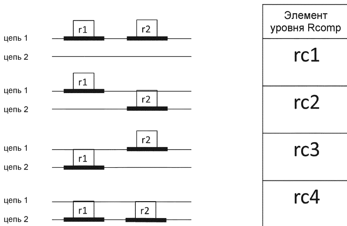
Фигура 10 - Четыре возможные комбинации считанных фрагментов, составляющих пары считанных фрагментов, и соответствующее кодирование на уровне rcomp.
