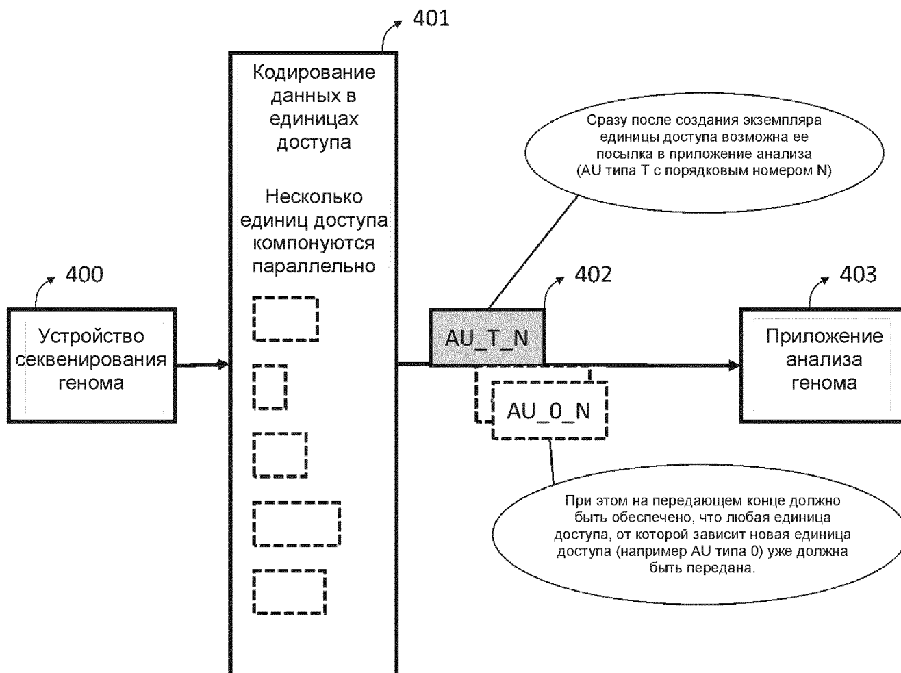
Фигура 41 - Структура данных на основе единиц доступа обеспечивает возможность анализа данных генома перед завершением процесса секвенирования.
