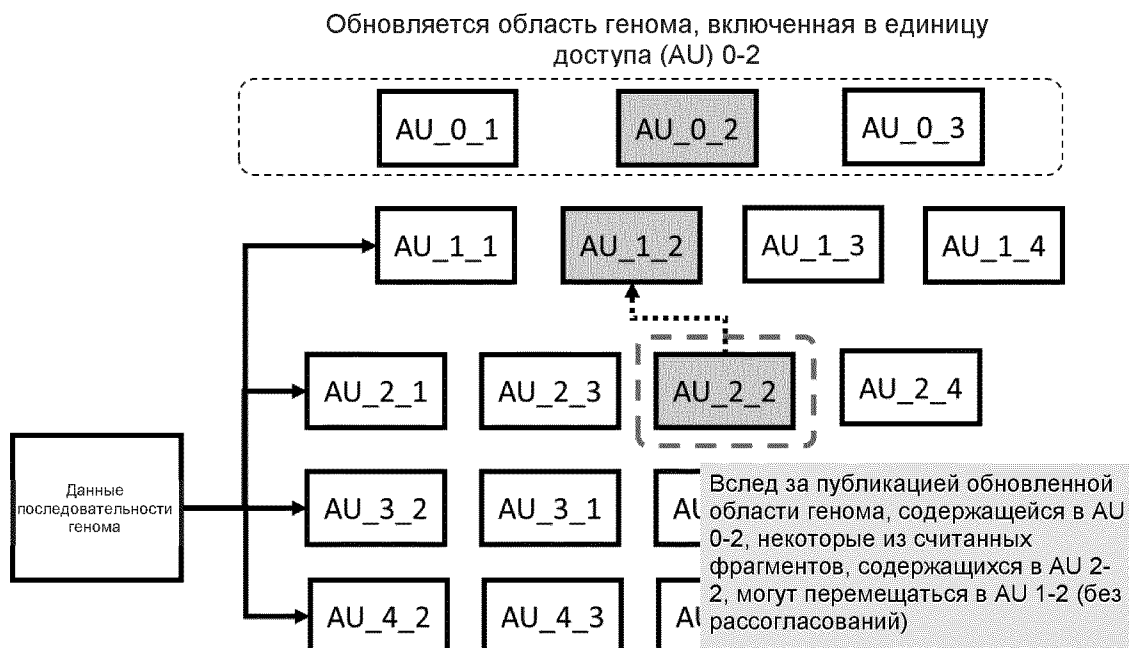
Фигура 44 - Транскодирование вследствие публикации новой референсной последовательности (генома).
