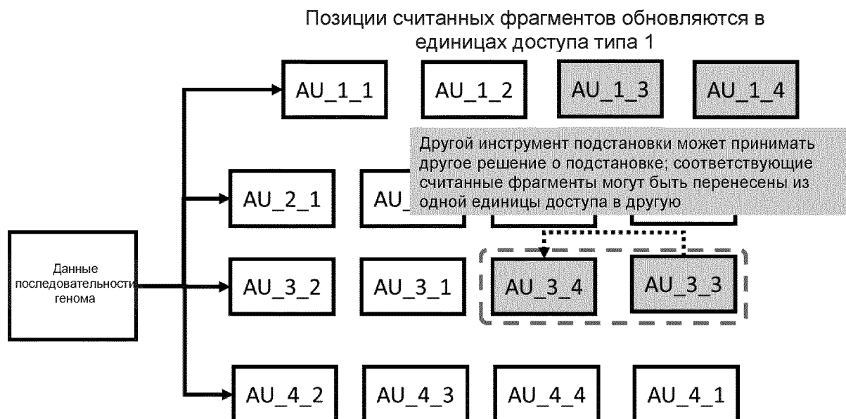
Фигура 46 – В случае обнаружения нового места подстановки (например, с меньшим количеством рассогласований) соответствующие считанные фрагменты могут перенесены из одной единицы доступа в другую того же типа.
