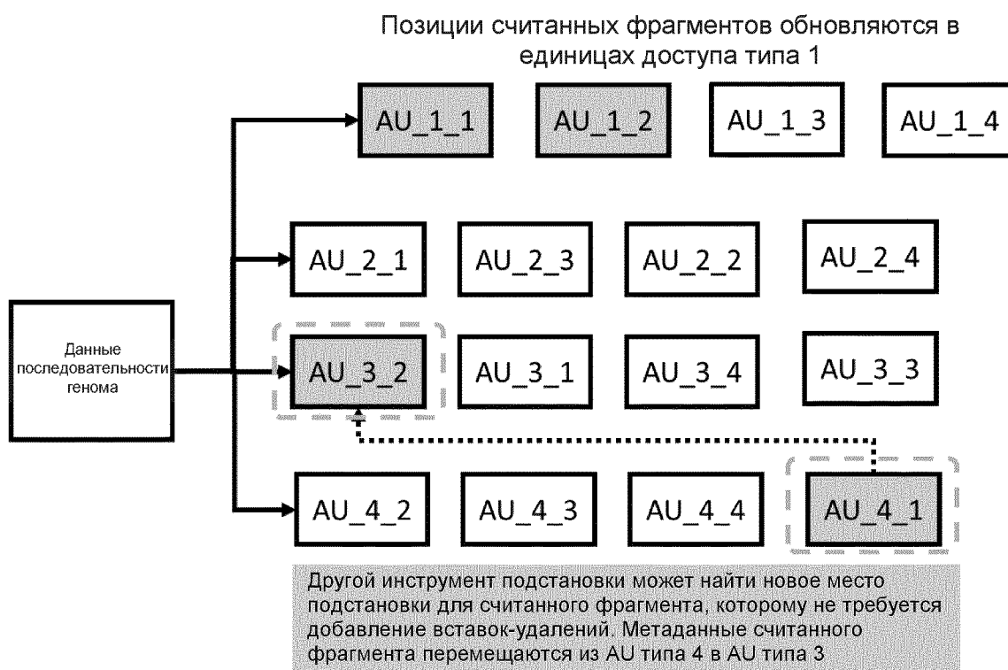
Фигура 45 - Считанные фрагменты, подставленные в новую область генома с повышенным качеством (например, без вставок-удалений) перемещаются из единицы доступа типа 4 в единицу доступа типа 3.
