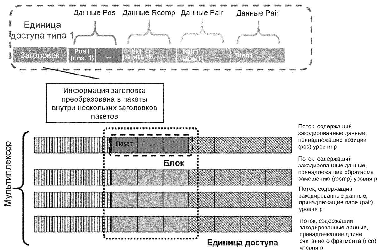
Фигура 27 - Единица доступа типа 1 преобразована в пакет и транспортирована в уплотненном формате данных генома.
