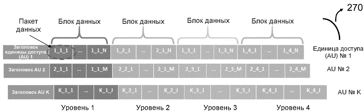
Фигура 28 - Единицы доступа образуются заголовками и уплотненными блоками, принадлежащими одному или более уровням однородных данных. Каждый блок может состоять из одного или более пакетов, содержащих действующие дескрипторы информации о геноме.
