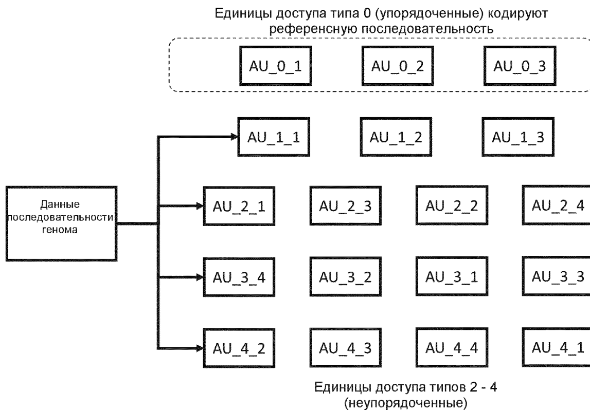
Фигура34 - Первые пять типов единиц доступа.
