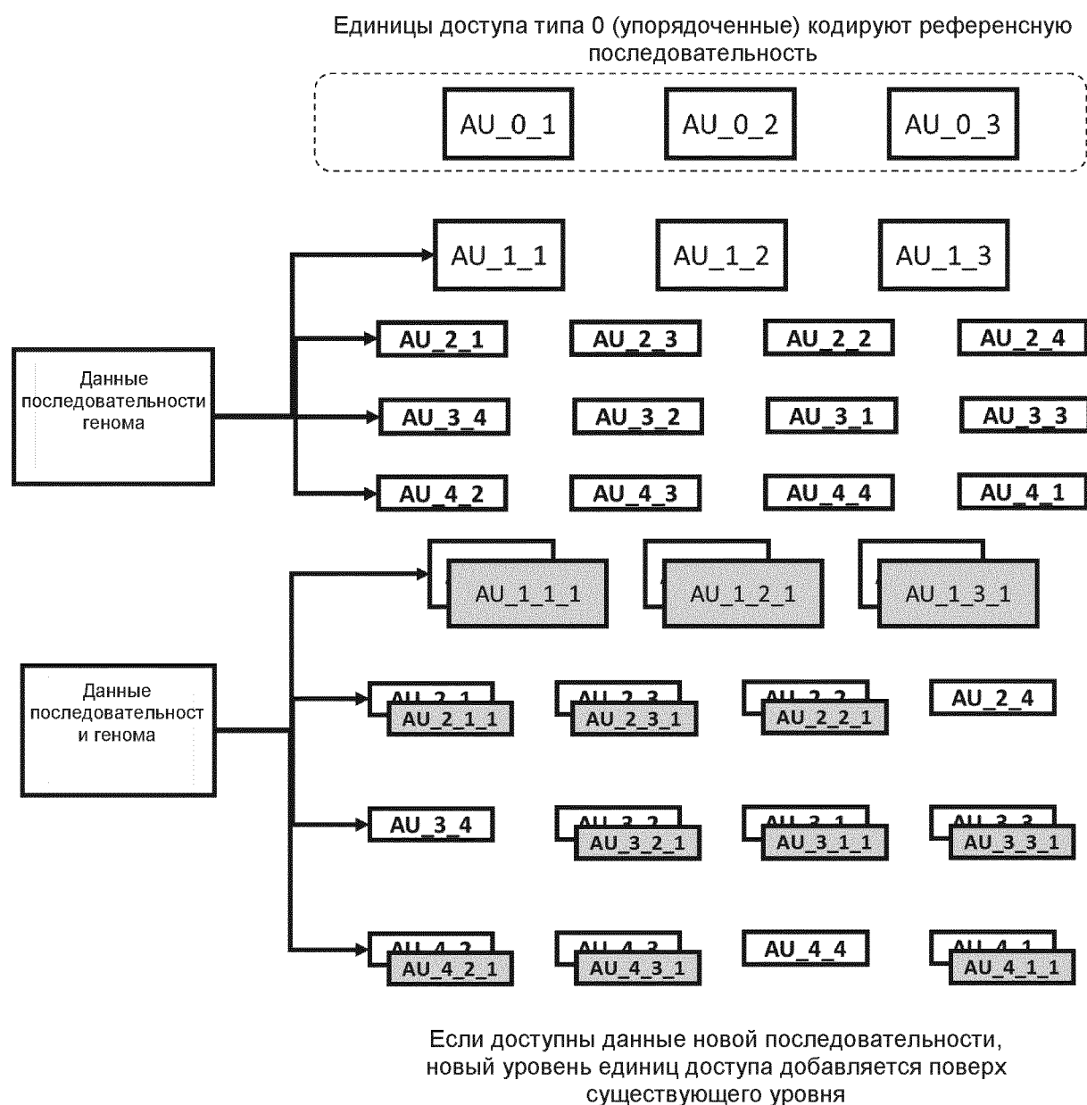
Фигура 40 - Когда доступны новые данные, поверх существующих данных создается новый уровень единиц доступа.
