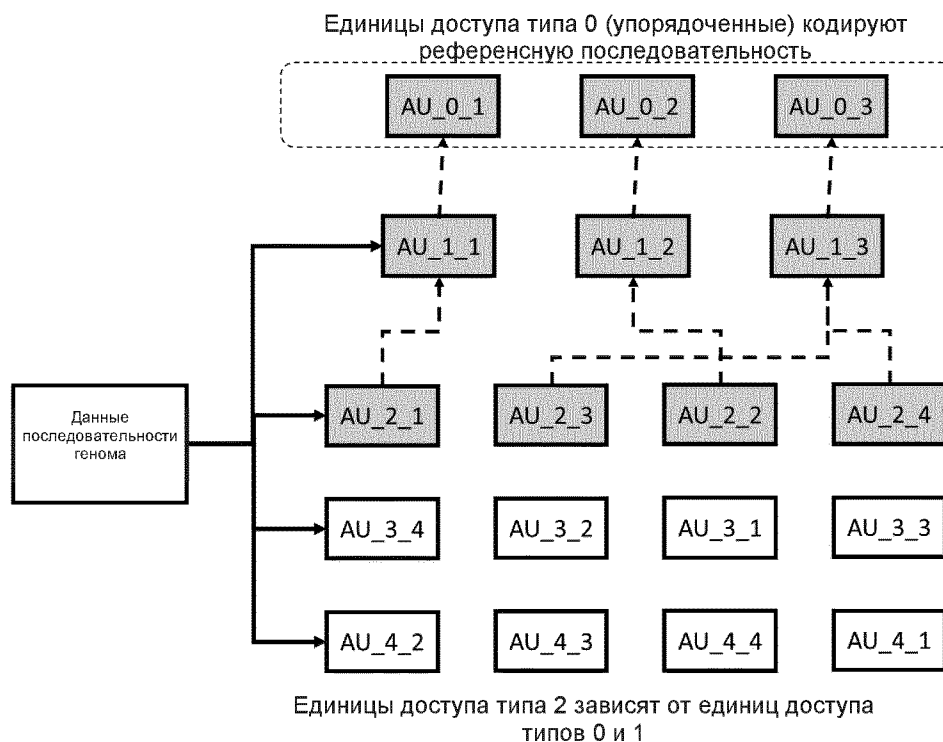
Фигура 36 - Единицы доступа типа 2 соотносятся с требующими декодирования единицами доступа типа 0 и 1.
