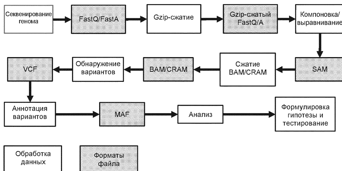
Фигура 1 - типовой конвейер обработки генома и форматы файла.
