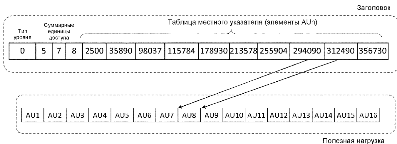
Фигура 24 – Пример таблицы местного указателя (LIT).
