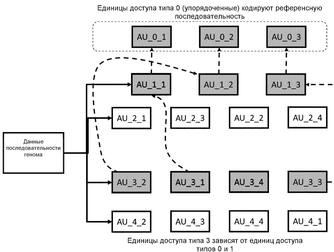
Фигура 37 - Единицы доступа типа 3 соотносятся с требующими декодирования единицами доступа типа 0 и 1.
