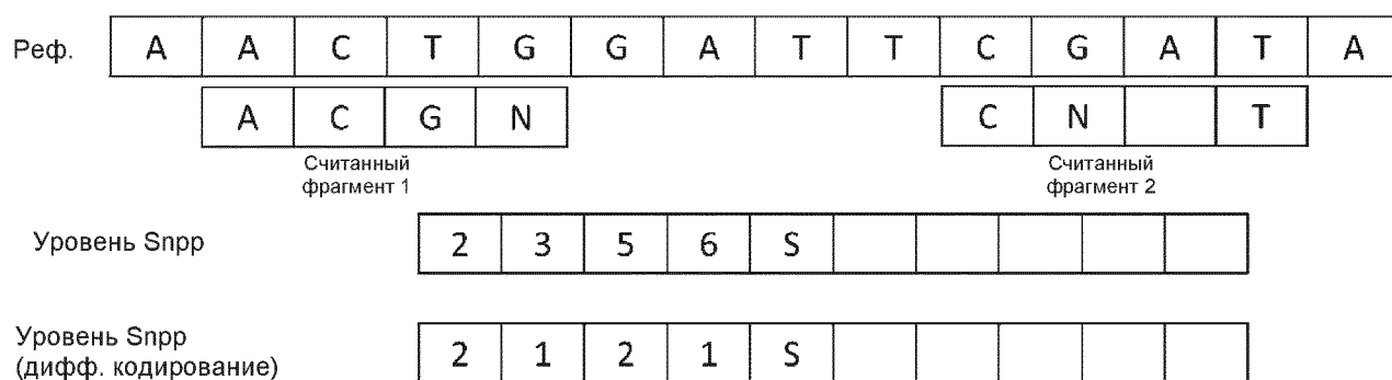
Фигура 13- Вычисление позиций замены в виде абсолютных или дифференциальных выражений.
