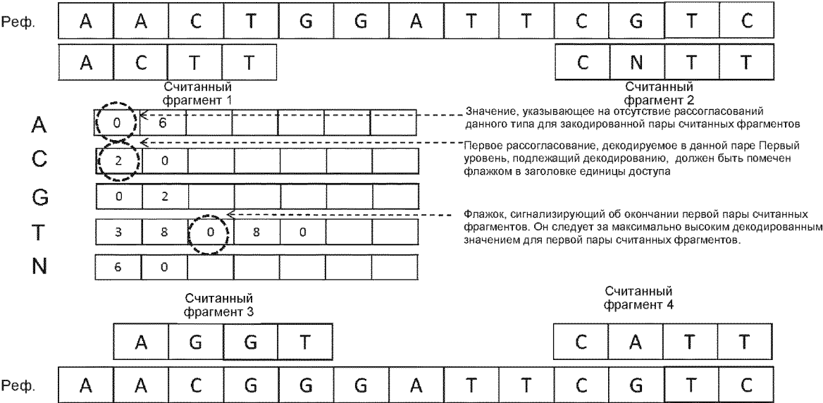
Фигура 17 – Альтернативная модель источника для замен, когда кодируются только позиции, но используется один уровень на тип замены.
