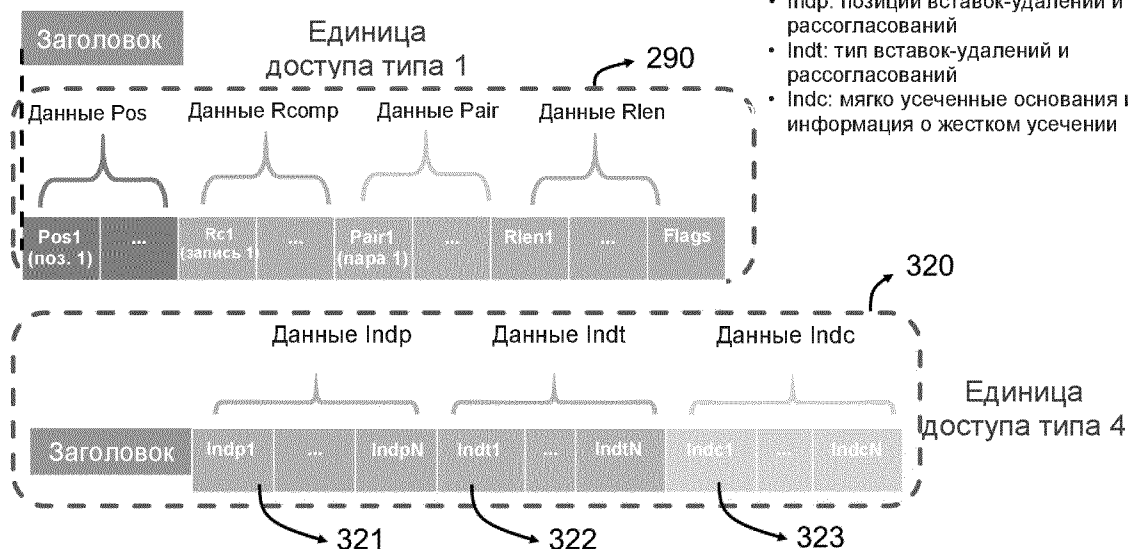
Фигура 33 - Единицы доступа типа 4 содержат данные, соотносимые с единицей доступа типа 1. В закодированных считанных фрагментах указываются позиции и типы рассогласования.
