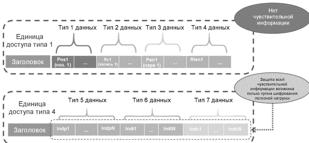
Фигура 47 – Избирательное шифрование может быть применено к единицам доступа типа 4 только при наличии в них чувствительной информации, требующей защиты.
