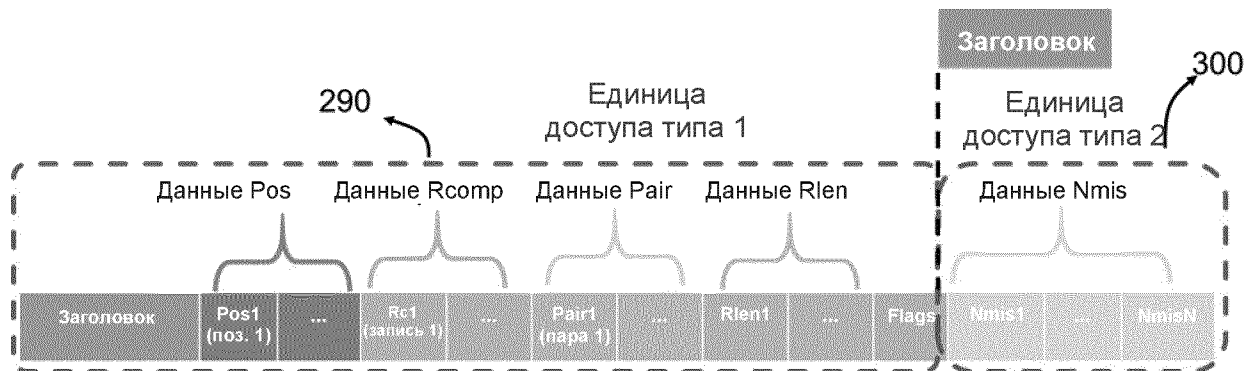
Фигура 31 - Единицы доступа типа 2 содержат данные, соотносимые с единицей доступа типа 1. Имеются позиции N в закодированных считанных фрагментах.
