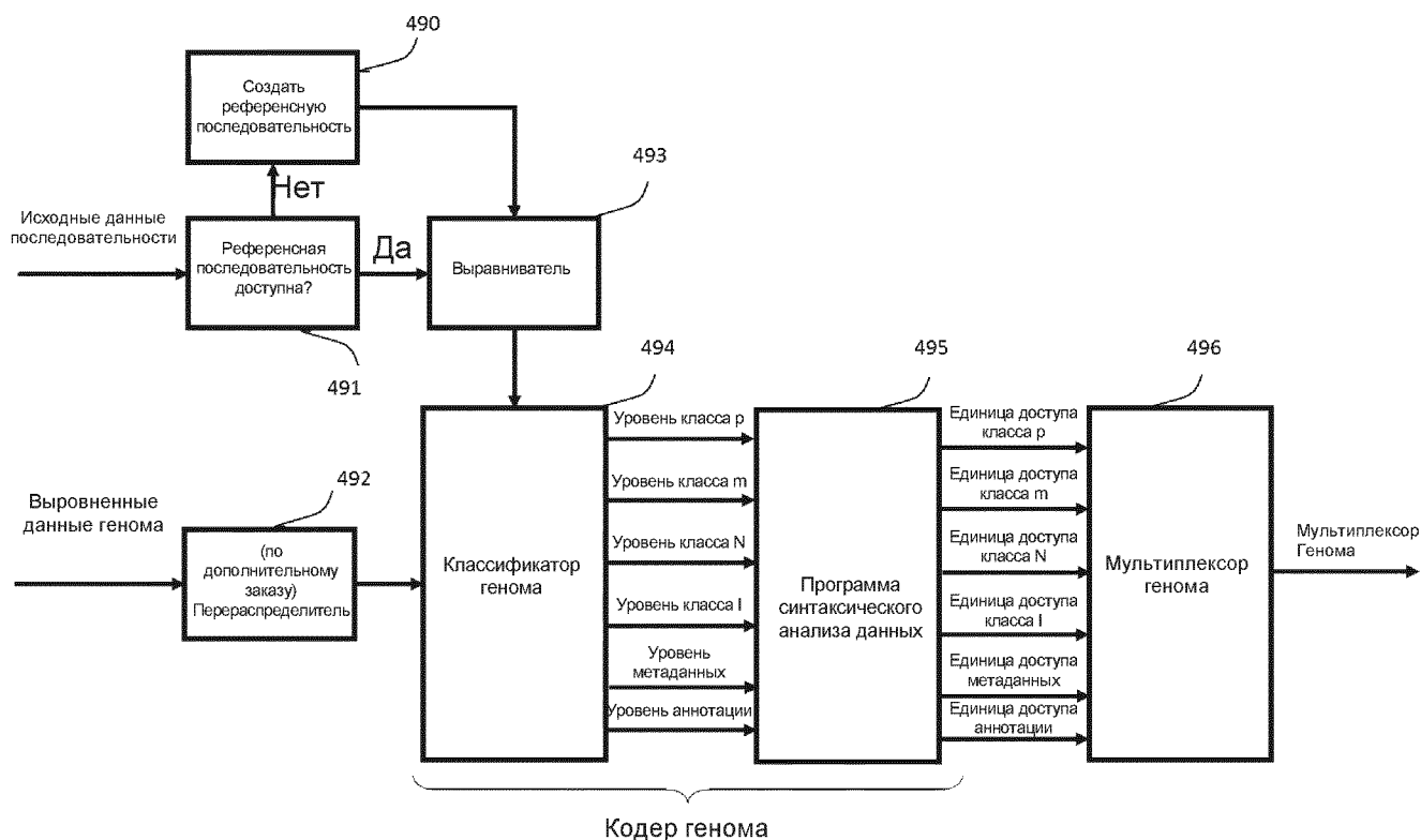
Фигура 48 - Кодер генома представляет собой первую ступень классификации данных и вторую ступень синтаксического анализа и кодирования данных. Этому может предшествовать выравнивание на референсной последовательности, сгенерированной внешними или внутренними средствами. Кодер генома может использовать выравниватели и вновь созданные компоненты программы для подготовки данных к кодированию.
