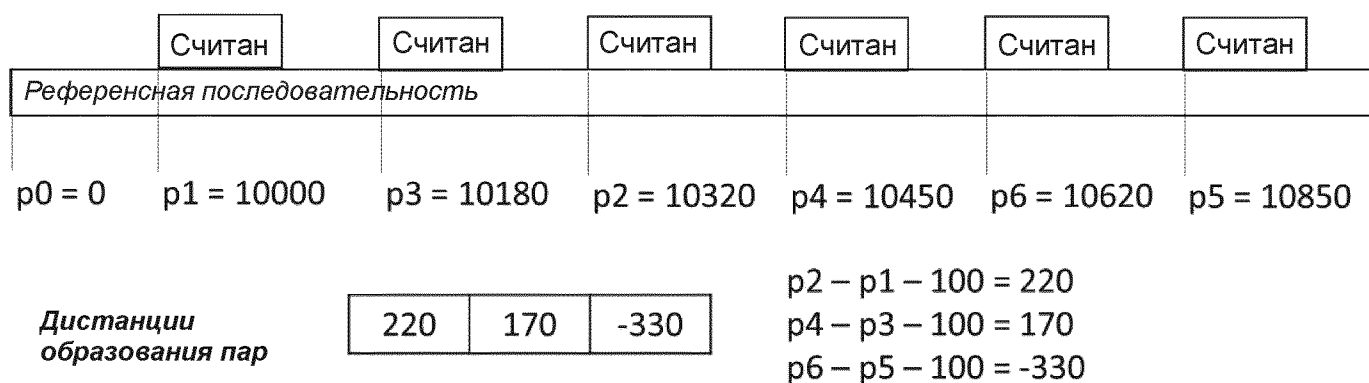
Фигура 5 - Вычисление расстояния образования пар для трех пар считанных фрагментов.
