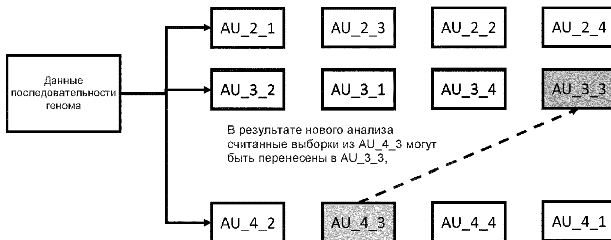
Фигура 42 - Для нового анализа, выполняемого на существующих данных, может понадобиться перемещение считанных фрагментов из единиц доступа типа 4 в единицу доступа типа 3.
