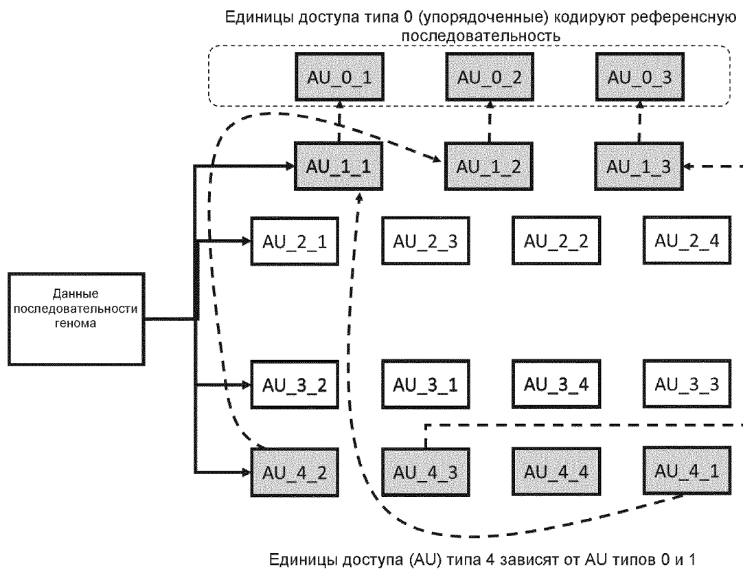
Фигура 38 - Единицы доступа типа 4 соотносятся с единицами доступа типа 1 для кодирования считанных фрагментов класса I.
