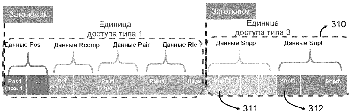
Фигура 32 - Единицы доступа типа 3 содержат данные, соотносимые с единицей доступа типа 1. В закодированных считанных фрагментах указываются позиции и типы рассогласования.
