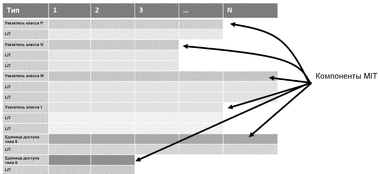
Фигура 25 – Функциональная взаимосвязь между таблицей Главного указателя и таблицами местных указателей.
