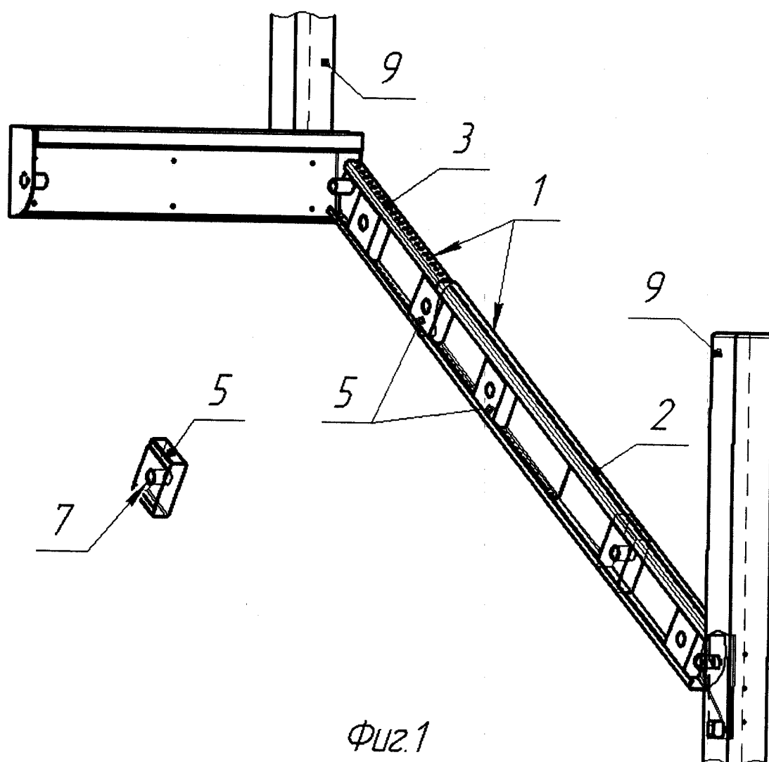
"Телескопическая тетива лестницы и узел крепления ступеней к телескопической тетиве лестницы"
