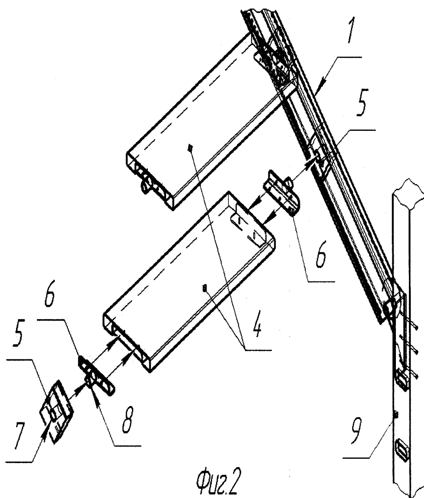
"Телескопическая тетива лестницы и узел крепления ступеней к телескопической тетиве лестницы"
