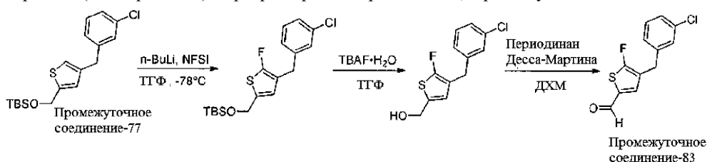
Пример 53. 4-(3-Хлорбензил)-5-фтортиофен-2-карбальдегид, Промежуточное соединение-83
