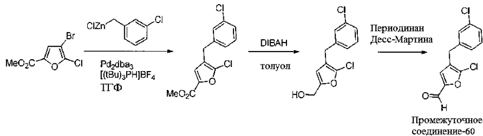
Пример 38. 5-Хлор-4-(3-хлорбензил)-2-фуральдегид, Промежуточное соединение-60
