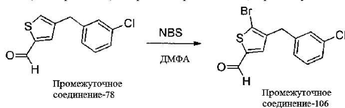
Пример 62. 5-Бром-4-(3-хлорбензил)тиофен-2-карбальдегид, Промежуточное соединение-106
