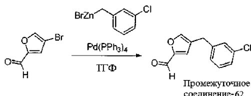
Пример 39. 4-(3-Хлорбензил)-2-фуриальдегид, Промежуточное соединение-62
