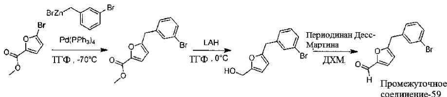
Пример 37. 5-(3-Бромбензил)-2-фуральдегид, Промежуточное соединение-59
