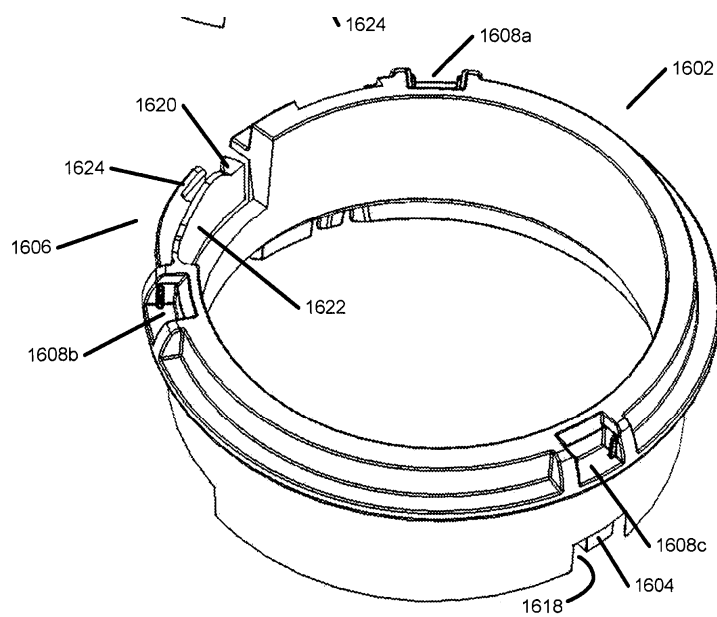
Фиг. 20В
