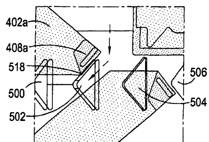
Фиг. 6А
