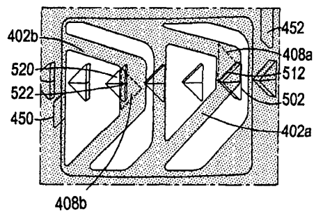
Фиг. 8А
