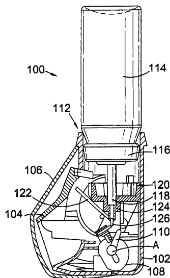
Фиг. 1
