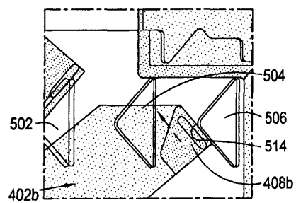
Фиг. 5С
