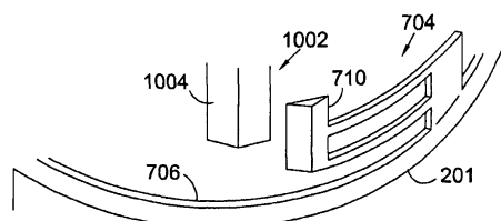
Фиг. 13D
