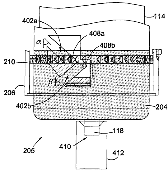
Фиг. 4А
