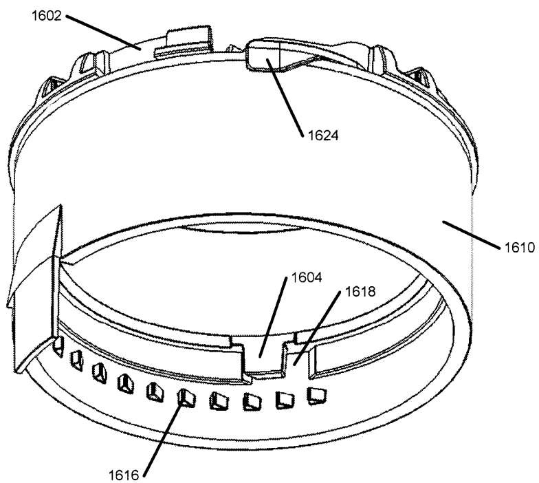
Фиг. 22В
