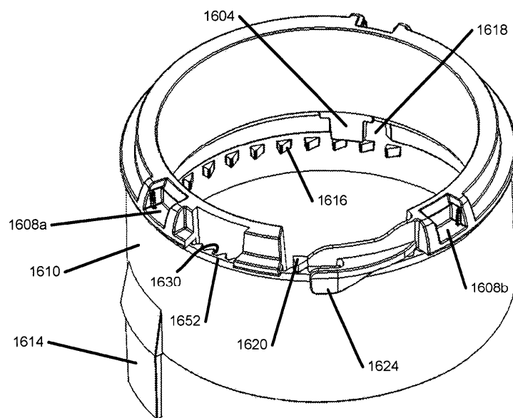
Фиг. 22А
