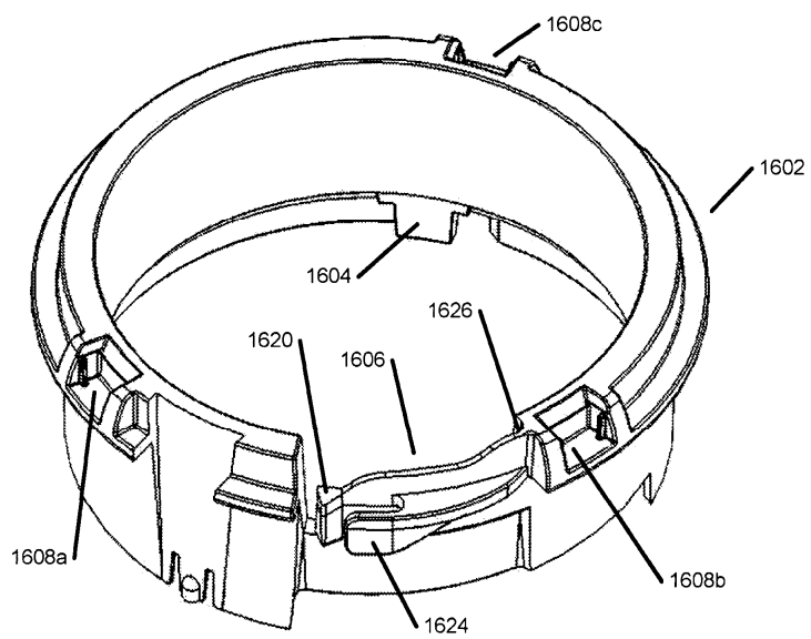
Фиг. 20А
