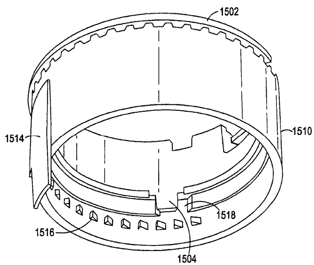
Фиг. 18С
