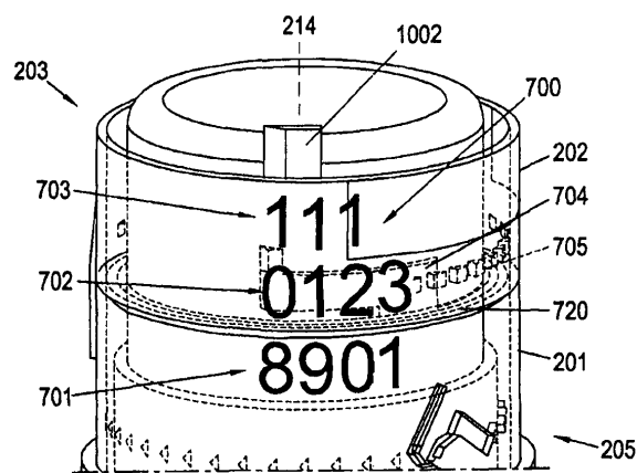
Фиг. 10
