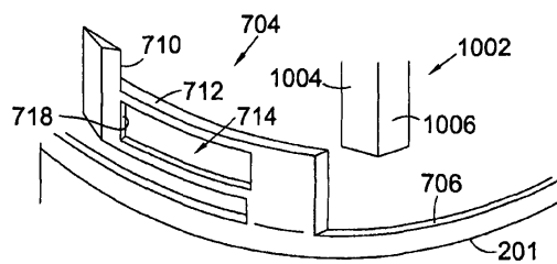
Фиг. 13А
