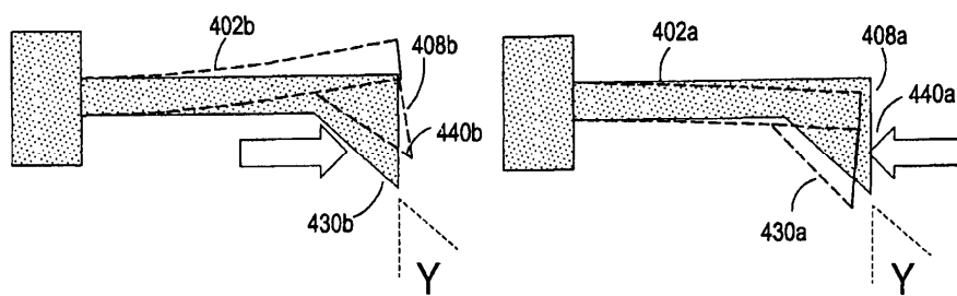
Фиг. 7B
