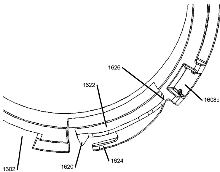
Фиг. 20С
