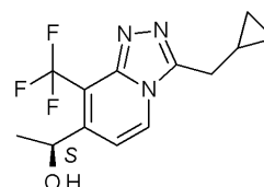
Промежуточное соединение 21c
