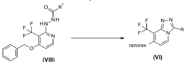
Схема реакции 5
