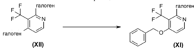
Схема реакции 8
