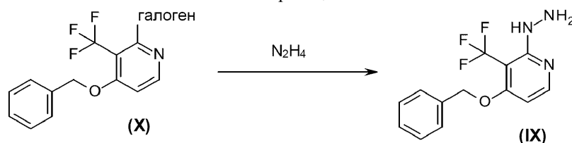
Схема реакции 7
