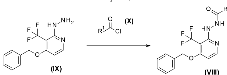
Схема реакции 6
