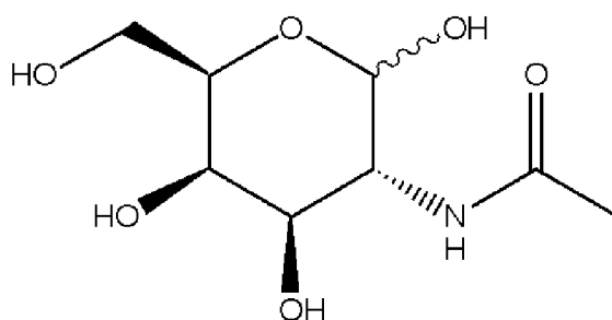
2-(Ацетиламино)-2-дезокс-D-галактопираноза
