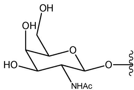
2-(Ацетиламино)-2-дезоксi-β-D-галактопираноза
