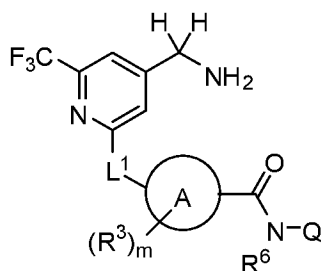
Формула (IV).
