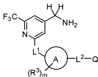
Формула (II).
