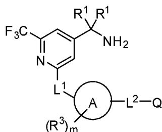
Формула (I)
