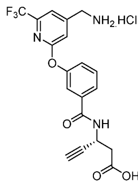
Соединение 1-223
