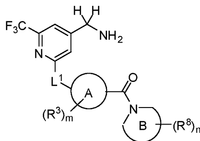
Формула (V)
