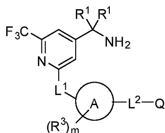
Формула (I),
