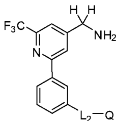
Формула (VII).
