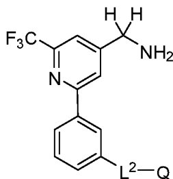
Формула (VII).
