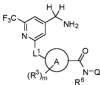
Формула (IV).
