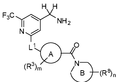
Формула (V),
