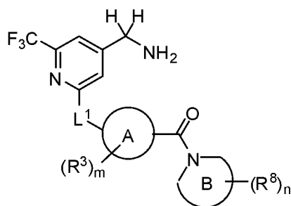
Формула (V)
