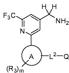
Формула (III).
