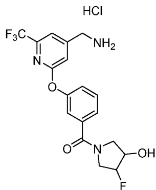
Рацемический транс-изомер
