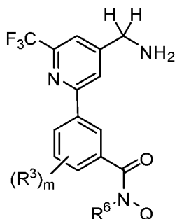
Формула (VIII).
