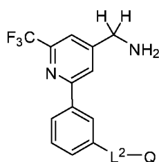
Формула (VII).
