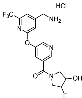
Рацемический транс-изомер
