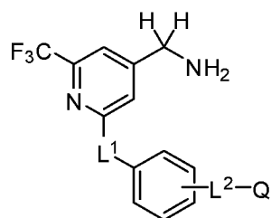
Формула (VI),
