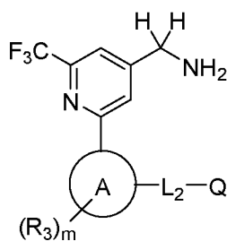
Формула (III).
