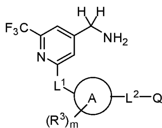
Формула (II).
