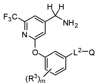
Формула (IX).
