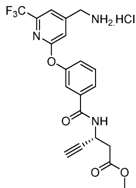
Соединение 1-222
