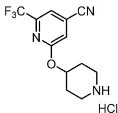
Int-G
