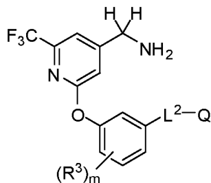
Формула (IX).
