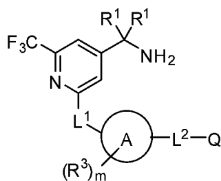
Формула (I),
