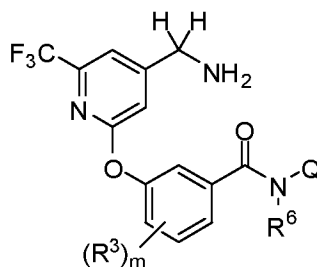
Формула (X).
