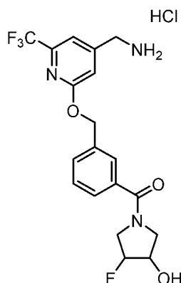
Рацемический транс-изомер
