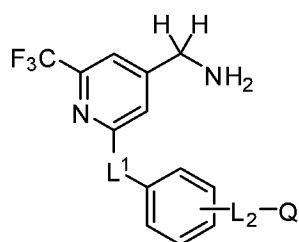
Формула (VI),
