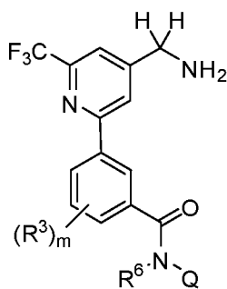
Формула (VIII).
