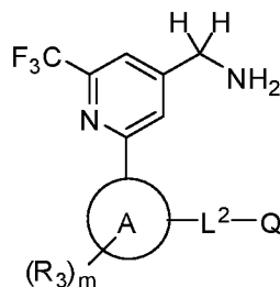
Формула (III).
