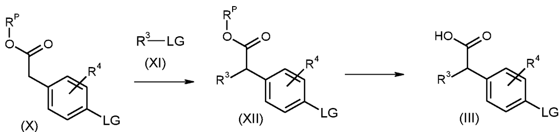
Схема 4: Получение производных замещенной фенилуксусной кислоты формулы (III) из алкилфенилацетатов формулы (X)
