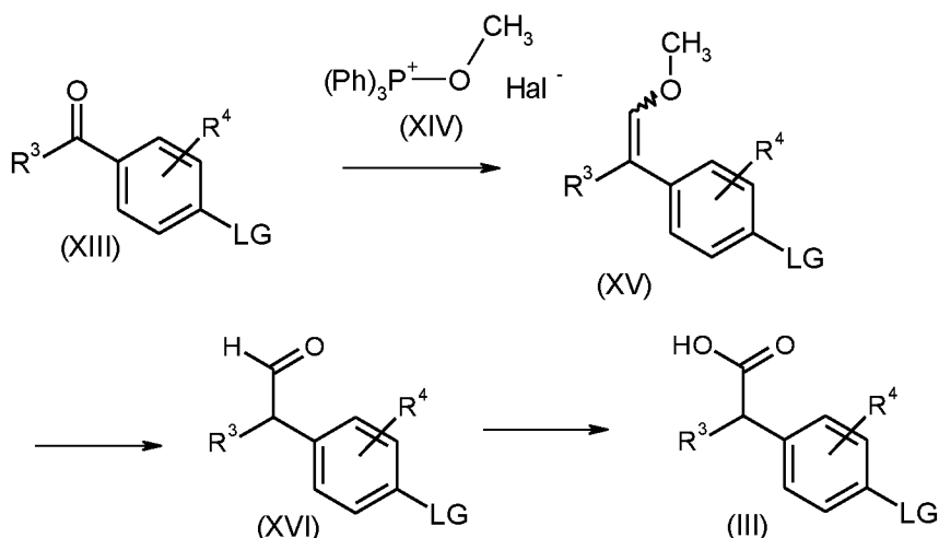
Схема 5: Получение производных замещенной фенилуксусной кислоты формулы (III) из кетонов формулы (XIII) 15
