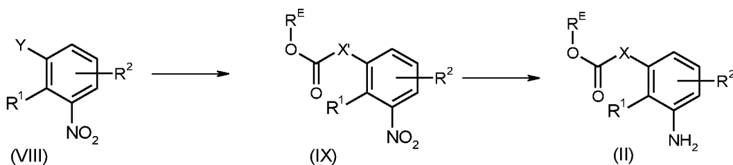
Схема 3: Получение анилиновых производных формулы (II) из предшественников формулы (VIII)
