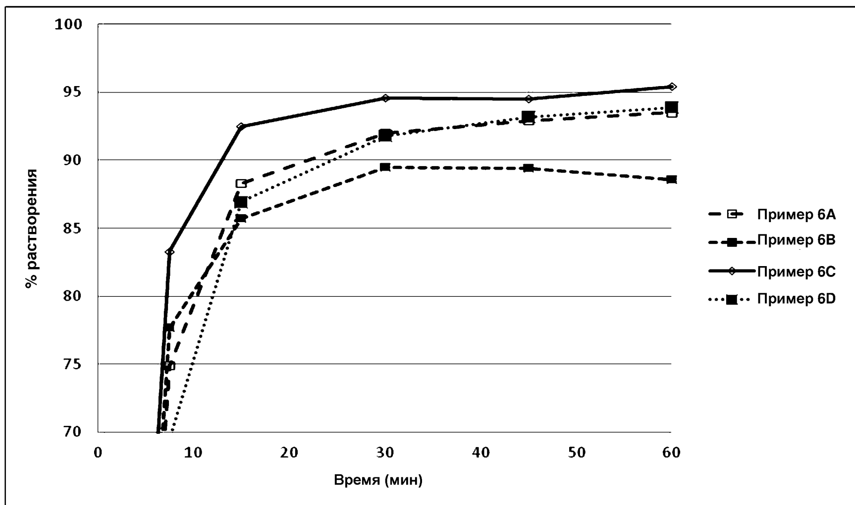
ФИГ. 3 –Профиль увеличенной растворимости для Примеров 6А, 6В, 6С и 6D (рН 6,8)
