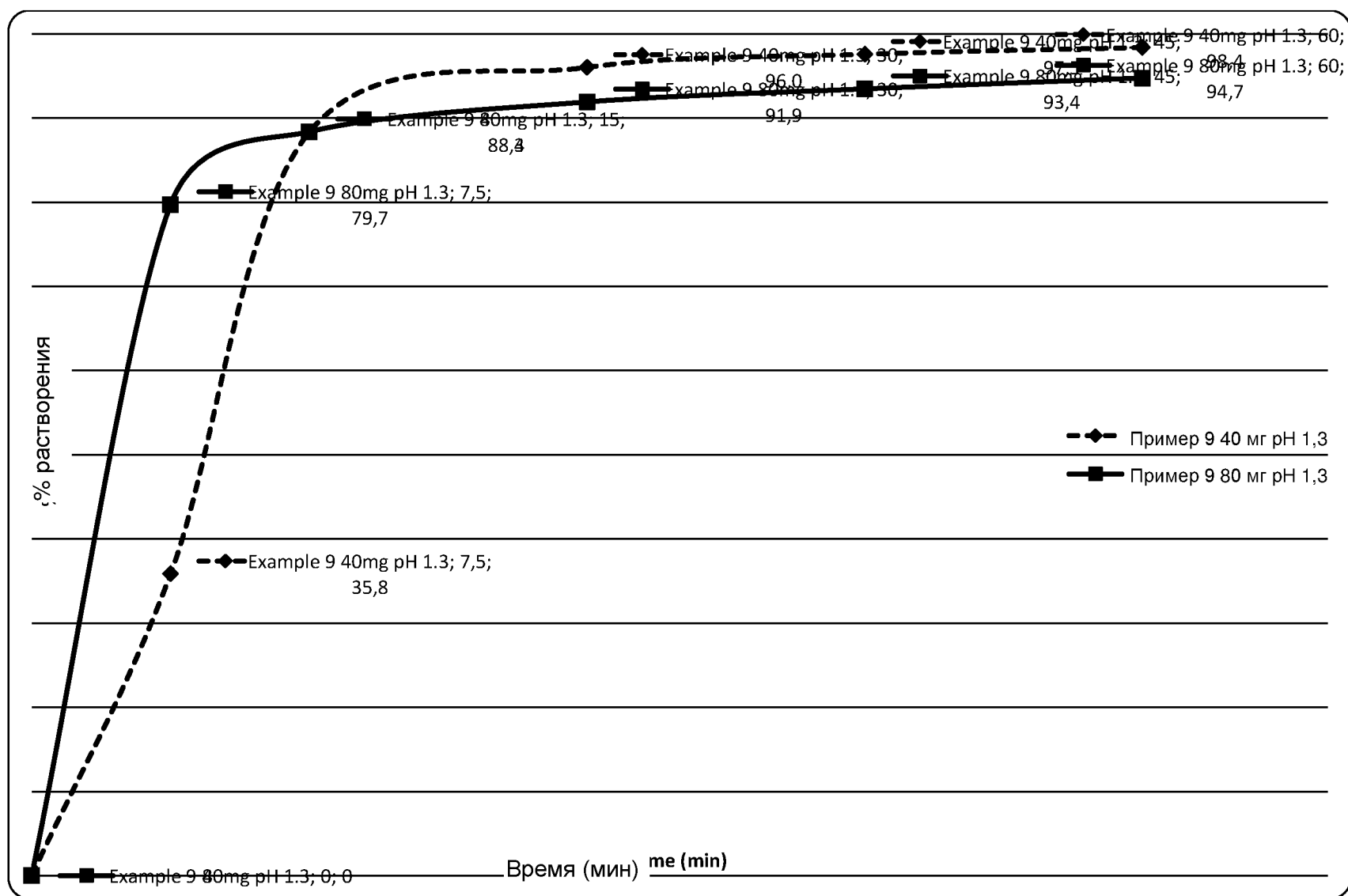
ФИГ. 6 –Профиль растворимости для Примера 9 (pH 1,3)
