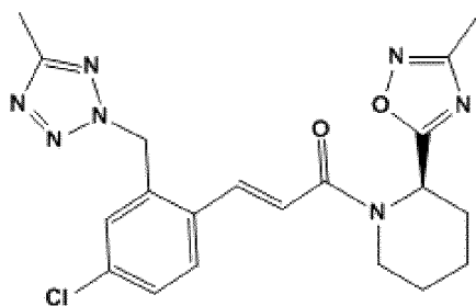
(R)-стереоизомер
