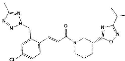
(R)- стереоизомер
