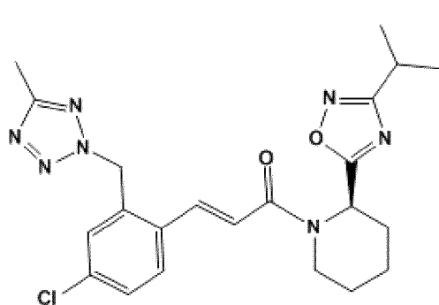
( R )- стереизомер
