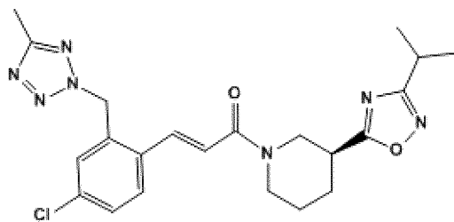
(S)- стереоизомер
