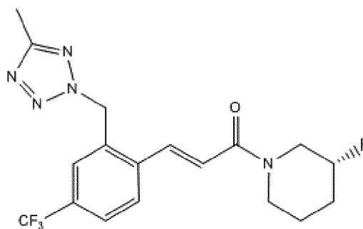
(R)- стереоизомер
