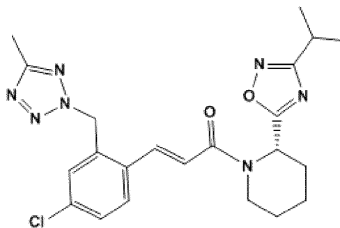
( S )- стереизомер
