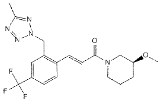
( S )-стереоизомер
