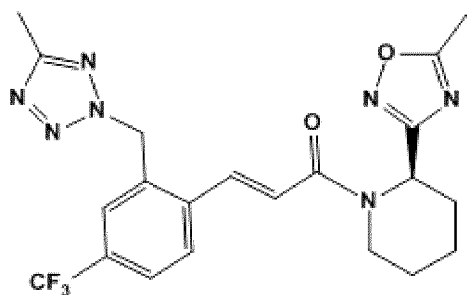
(R) -стереоизомер
