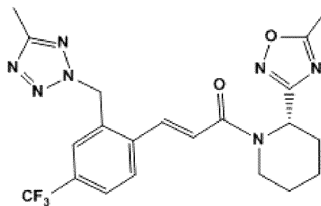
(S) -стереоизомер
