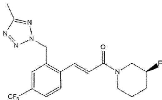
(S)-стереоизомер
