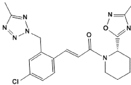
(S)-стереоизомер
