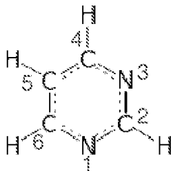
Пиримидин .
