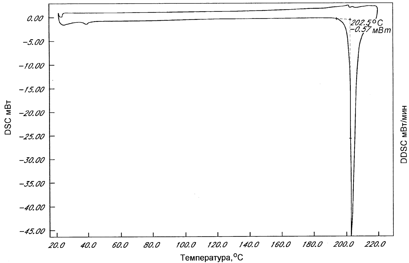
Фиг. 2 Результаты цифровой сканирующей калориметрии для Формы I
