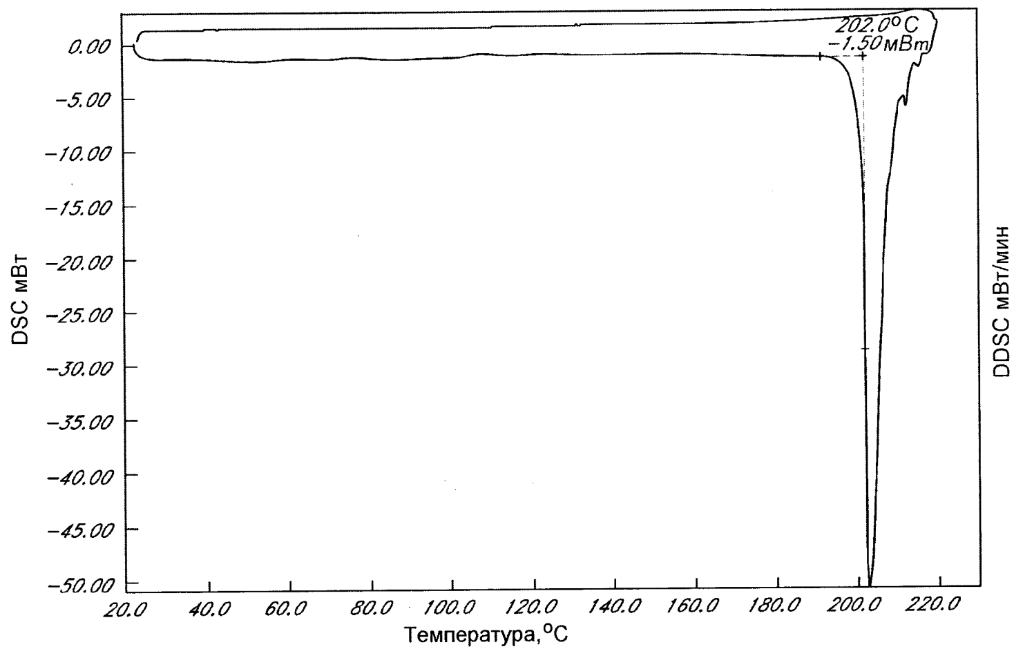
Фиг. 7 Результаты цифровой сканирующей калориметрии для Формы II
