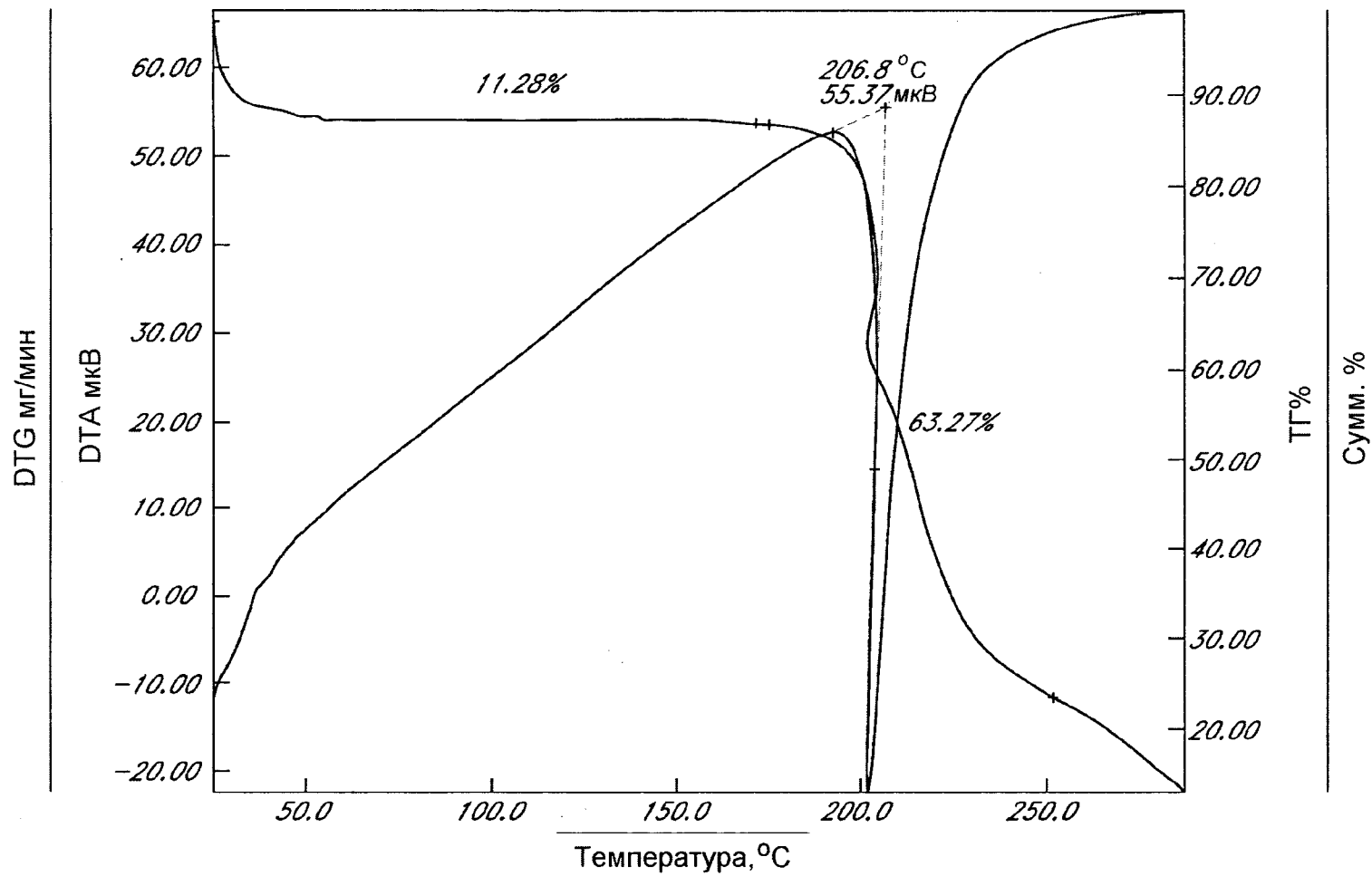
Фиг. 3 Термогравиметрический гравиметрический/дифференциальный термический анализ Формы I
