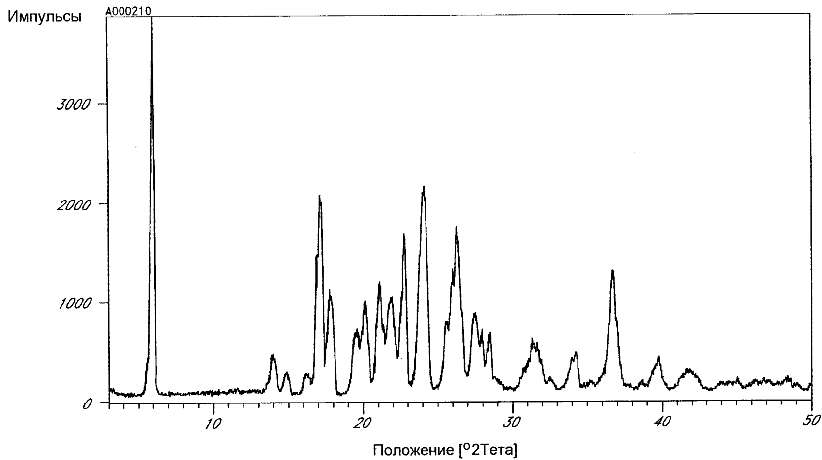
Порошковая рентгеновская дифрактограмма Формы II
