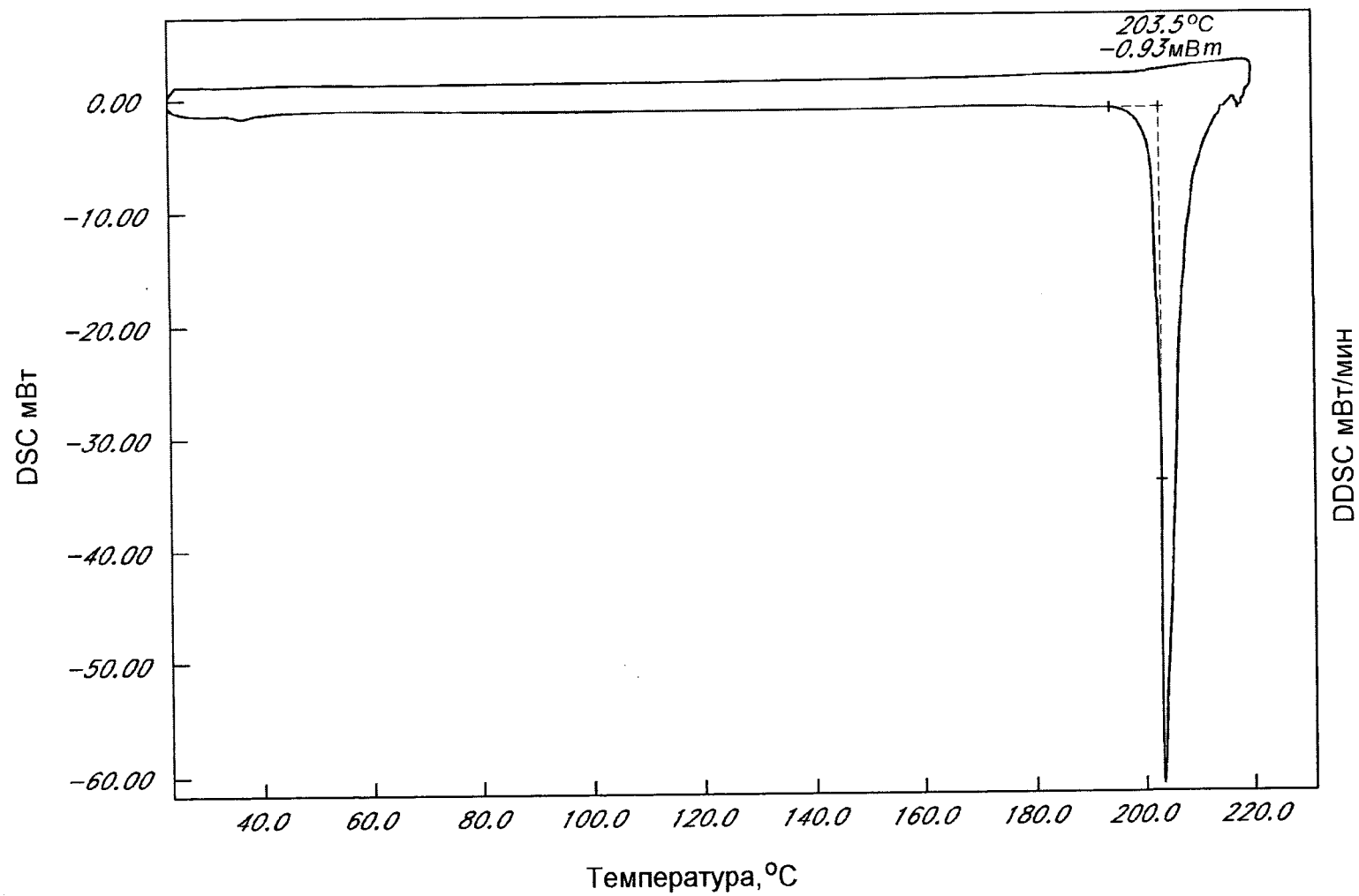
Фиг. 12 Результаты цифровой сканирующей калориметрии для Формы III
