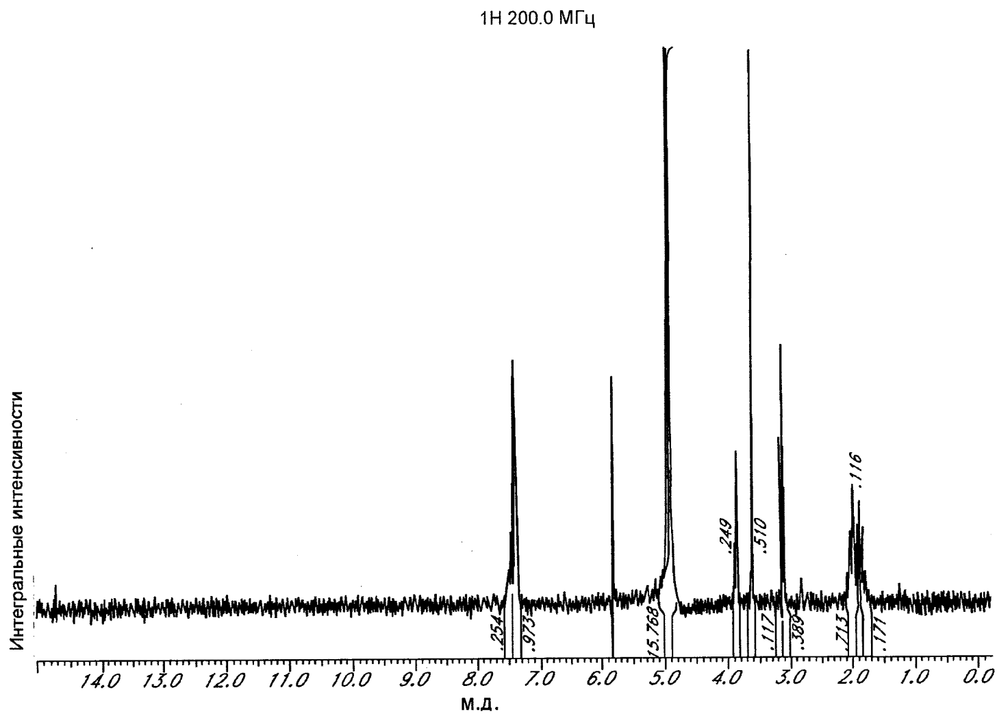
Фиг. 4 Спектр ^1\text{H} -ядерного магнитного резонанса, полученный для Формы I
