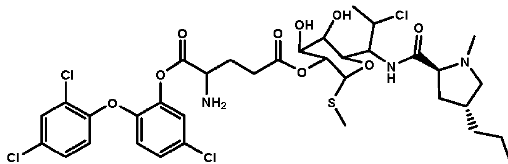
Клиндамицин-триклозан с глутаминовой кислотой
