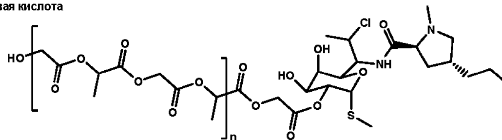
Конъюгат клиндамицин-гликолевая кислота-ПМГК
