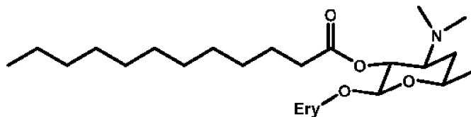
Конъюгат эритромицин-лауриновая кислота
