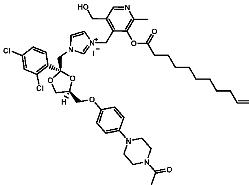
Конъюгат кетоконазол-пиридоксин- ундециленовая кислота
