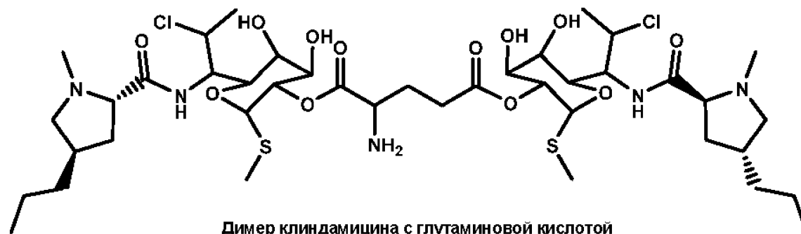
Димер клиндамицина с глутаминовой кислотой
