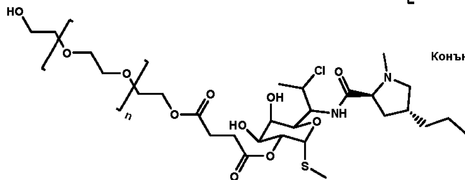
Конъюгат клиндамицин-янтарная кислота-ПЭГ
