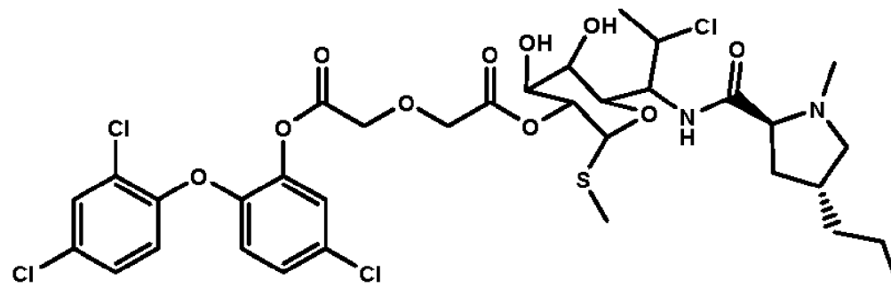
Клиндамицин-триклозан с оксидиуксусной кислотой
