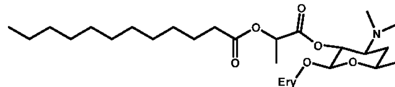
Конъюгат эритромицин-молочная кислота- лауриновая кислота
