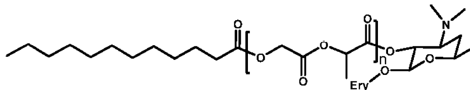
Конъюгат лауриновая кислота-СМГК-эритроамицин
