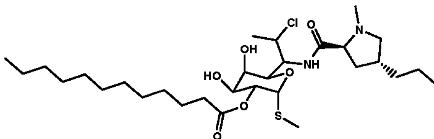
Конъюгат клиндамицин-лауриновая кислота
